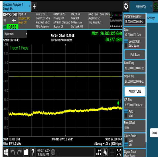
NTVN-N7-PC3-15-20-M-DFT-QPSK-Edge_1RB_Left-Ant1-
