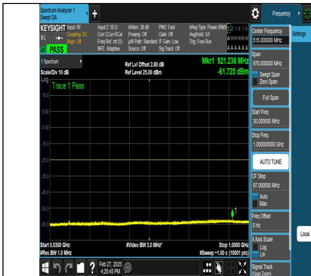
NTNV-N7-PC3-15-5-L-DFT-QPSK-Edge 1RB Left-Ant1-PASS
