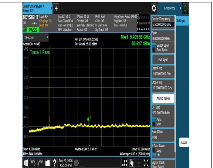
NTNV-N7-PC3-15-5-L-DFT-QPSK-Edge 1RB Left-Ant1-PASS
