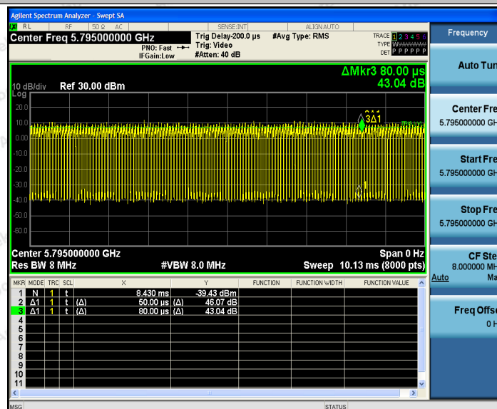
11N40SISO_Ant2_5795
