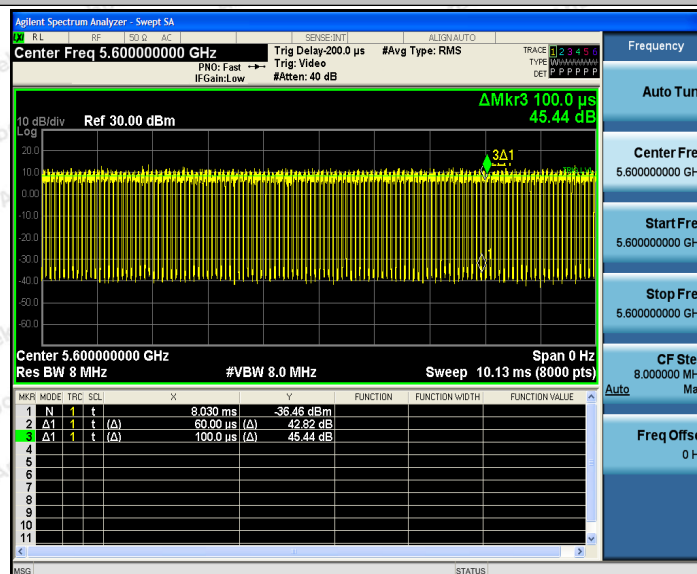
11A_Ant2_5600
