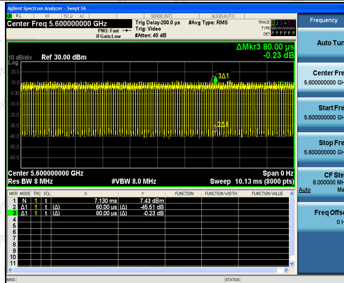
11A_Ant2_5600
