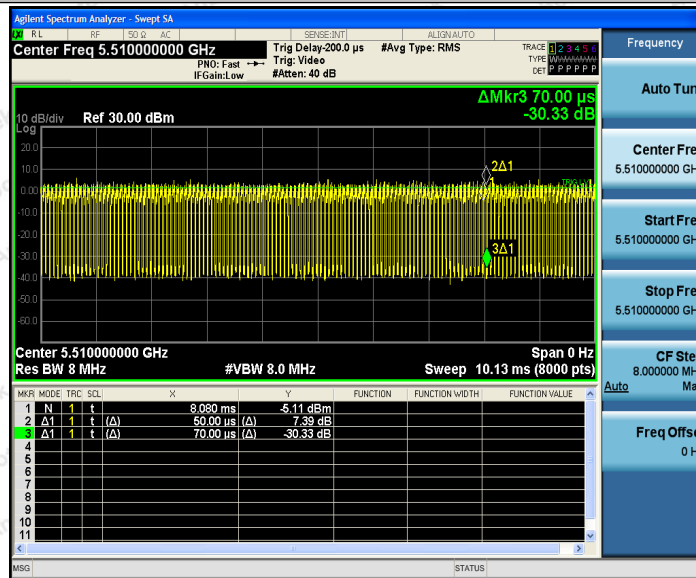
11N40SISO_Ant2_5510
