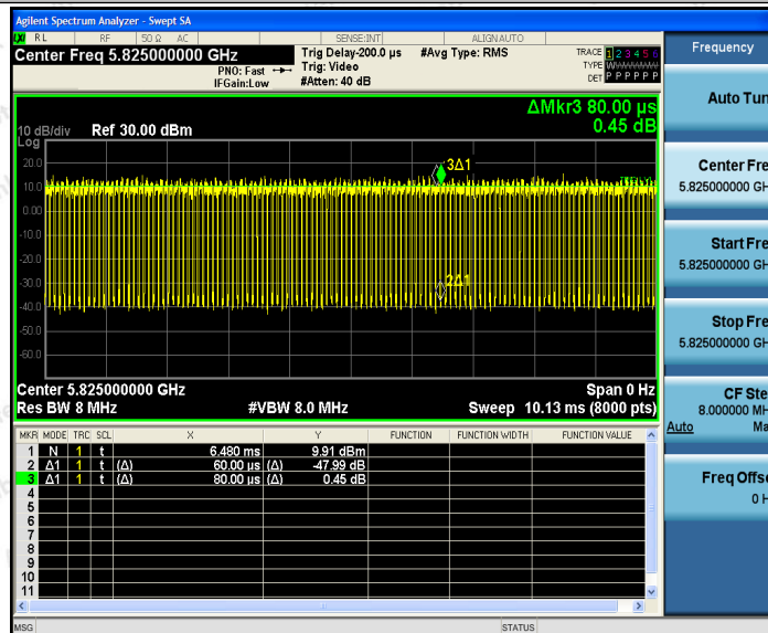
11A_Ant2_5825
