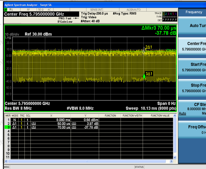
11N40SISO_Ant2_5795
