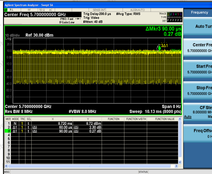
11N20SISO_Ant2_5700
