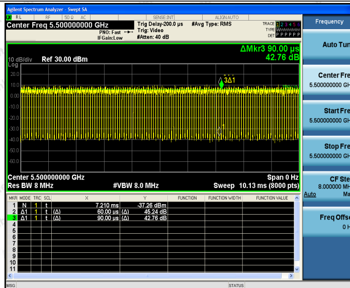
11A_Ant2_5500
