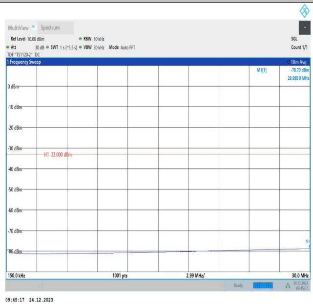
2-2-20MHz-10MHz-QPSK-QPSK-18700-18844-1RB#0-1RB#4 9-0.15~30MHz-PASS
