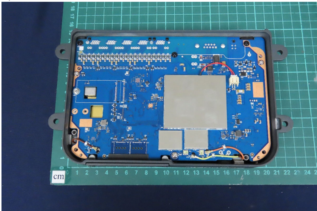
(40) EUT Photo
