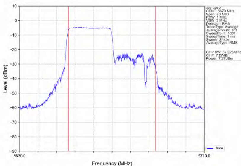
802.11ax(HE40) HCH 5670MHz RU242 Left Ant2 NTNv
