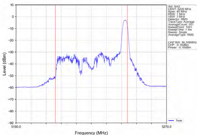
802.11ax(HE40) HCH 5230MHz RU26 Right Ant2 NTNv
