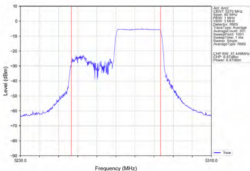
802.11ax(HE40) LCH 5270MHz RU242 Right Ant2 NTVN
