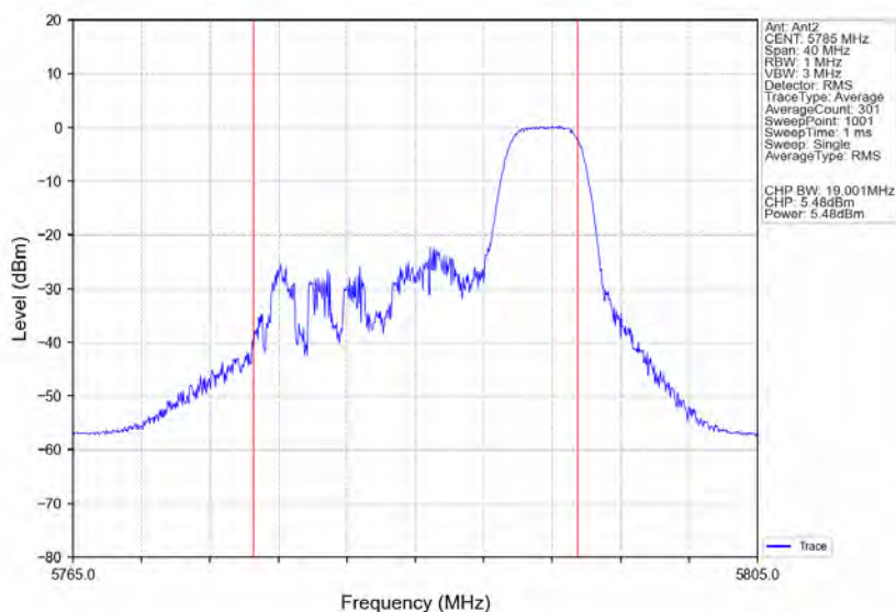
802.11ax(HE20) MCH 5785MHz RU52 Right Ant2 NTN
