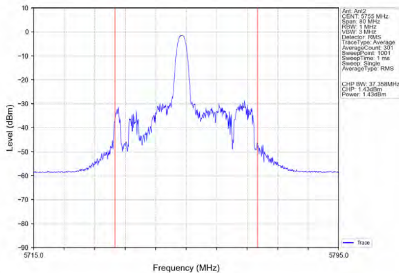
802.11ax(HE40) LCH 5755MHz RU26 Mid Ant2 NTN
