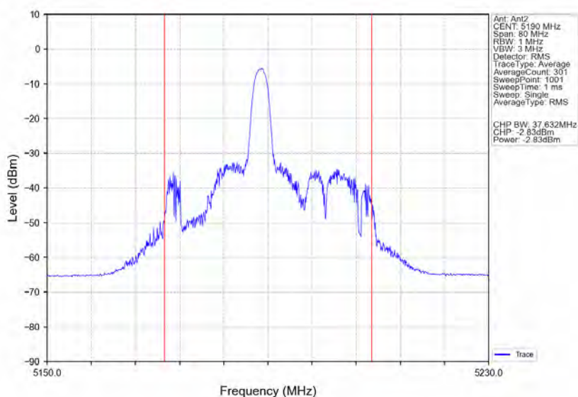
802.11ax(HE40) LCH 5190MHz RU26 Mid Ant2 NTN
