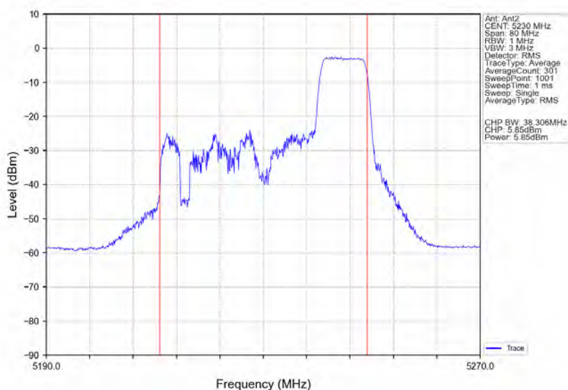
802.11ax(HE40) HCH 5230MHz RU106 Right Ant2 NTVN
