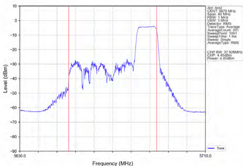
802.11ax(HE40) HCH 5670MHz RU106 Right Ant2 NTV
