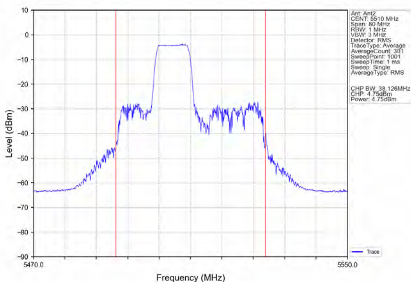
802.11ax(HE40) LCH 5510MHz RU106 Mid Ant2 NTNv
