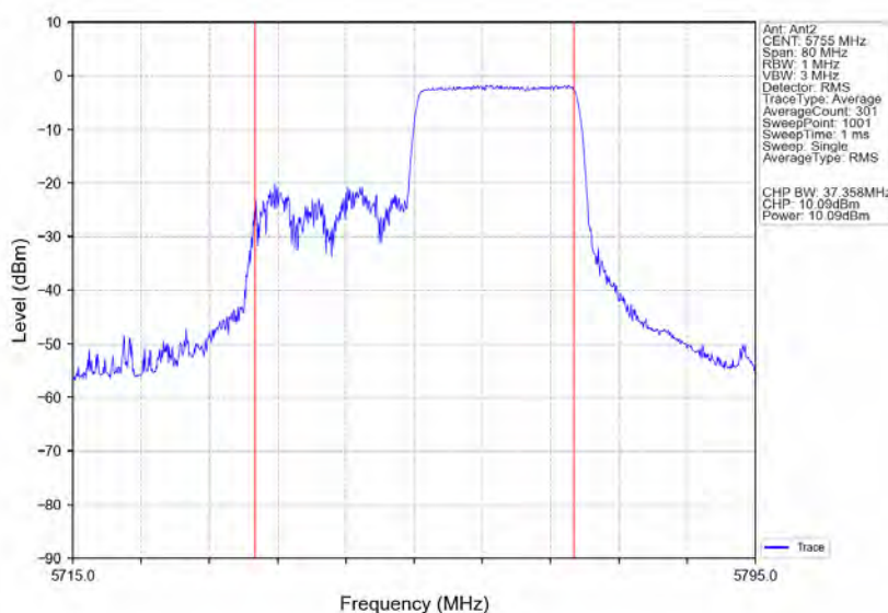
802.11ax(HE40) LCH 5755MHz RU242 Right Ant2 NTV
