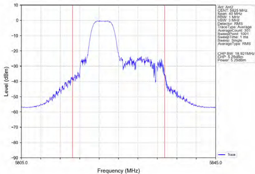
802.11ax(HE20) HCH 5825MHz RU52 Mid Ant2 NTNv
