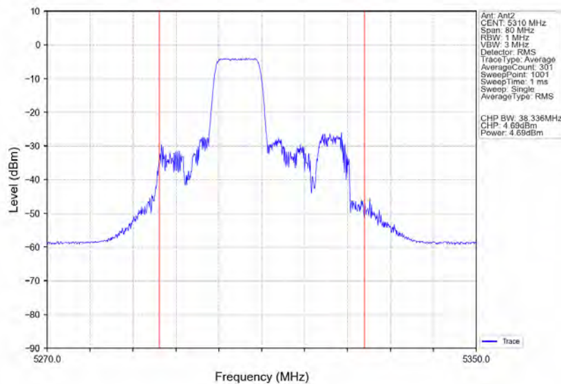
802.11ax(HE40) HCH 5310MHz RU106 Mid Ant2 NTNv
