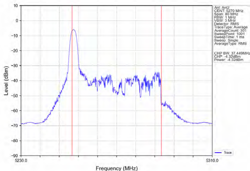
802.11ax(HE40) LCH 5270MHz RU26 Left Ant2 NTN
