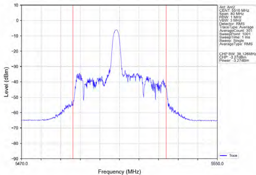
802.11ax(HE40) LCH 5510MHz RU26 Mid Ant2 NTNv
