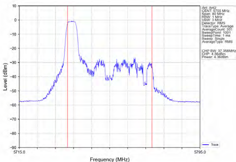
802.11ax(HE40) LCH 5755MHz RU52 Left Ant2 NTN
