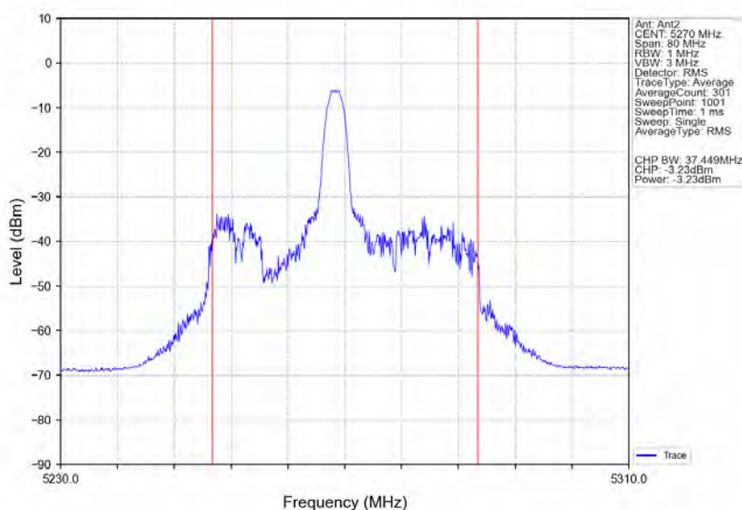
802.11ax(HE40) LCH 5270MHz RU26 Mid Ant2 NTNv
