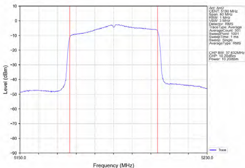
802.11ax(HE40) LCH 5190MHz RU484 Left Ant2 NTNv
