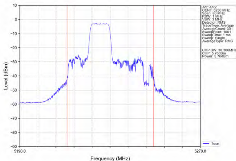
802.11ax(HE40) HCH 5230MHz RU106 Mid Ant2 NTNv
