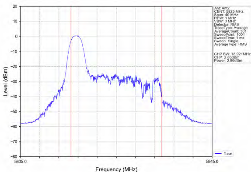
802.11ax(HE20) HCH 5825MHz RU26 Left Ant2 NTN
