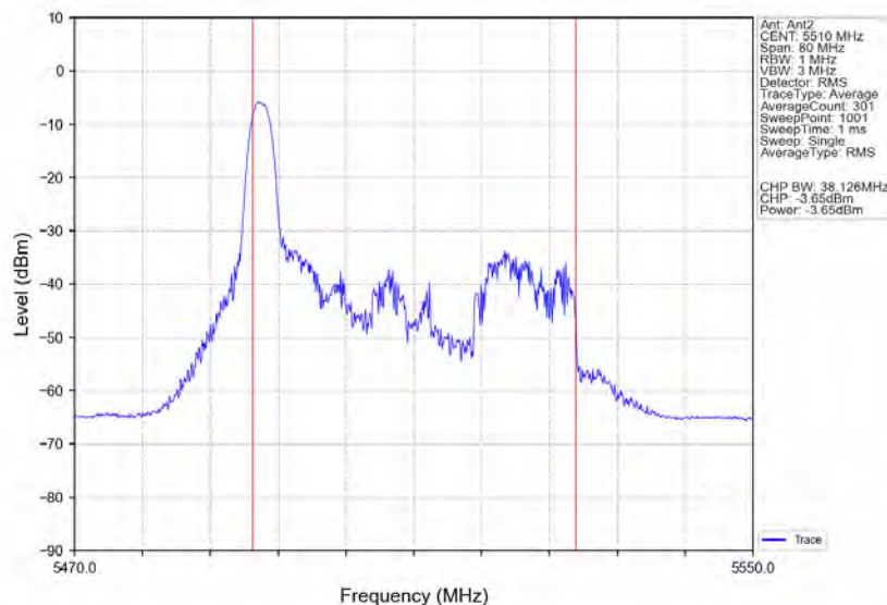
802.11ax(HE40) LCH 5510MHz RU26 Left Ant2 NTN
