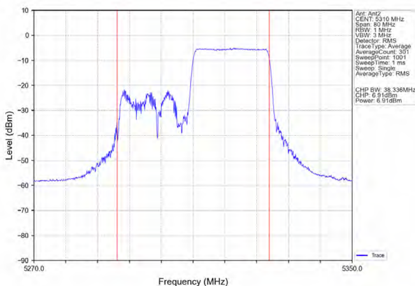
802.11ax(HE40) HCH 5310MHz RU242 Right Ant2 NTV
