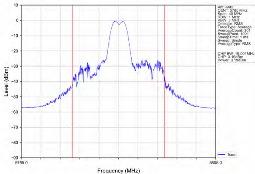
802.11ax(HE20) MCH 5785MHz RU26 Mid Ant2 NTN
