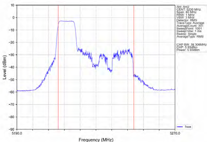
802.11ax(HE40) HCH 5230MHz RU106 Left Ant2 NTNv
