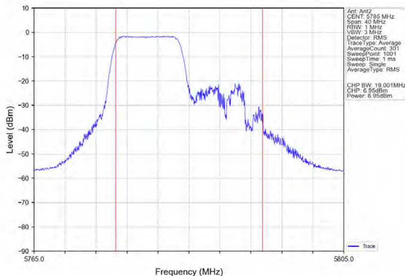
802.11ax(HE20) MCH 5785MHz RU106 Left Ant2 NTNv
