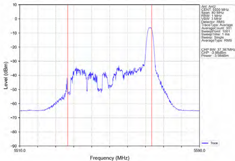
802.11ax(HE40) MCH 5550MHz RU26 Right Ant2 NTN
