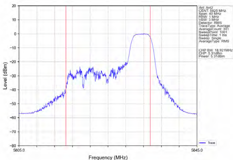
802.11ax(HE20) HCH 5825MHz RU52 Right Ant2 NTNv
