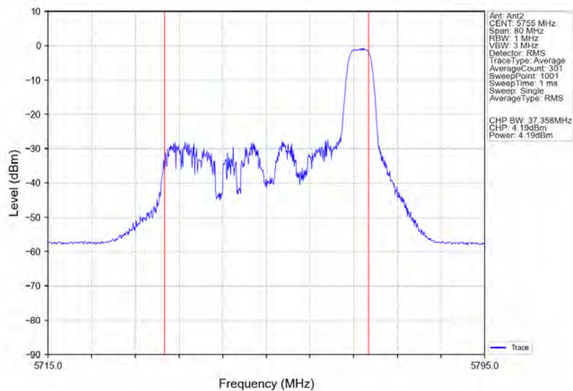
802.11ax(HE40) LCH 5755MHz RU52 Right Ant2 NTNv
