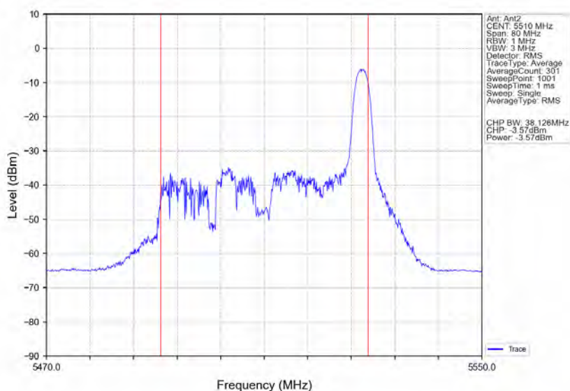
802.11ax(HE40) LCH 5510MHz RU26 Right Ant2 NTNv
