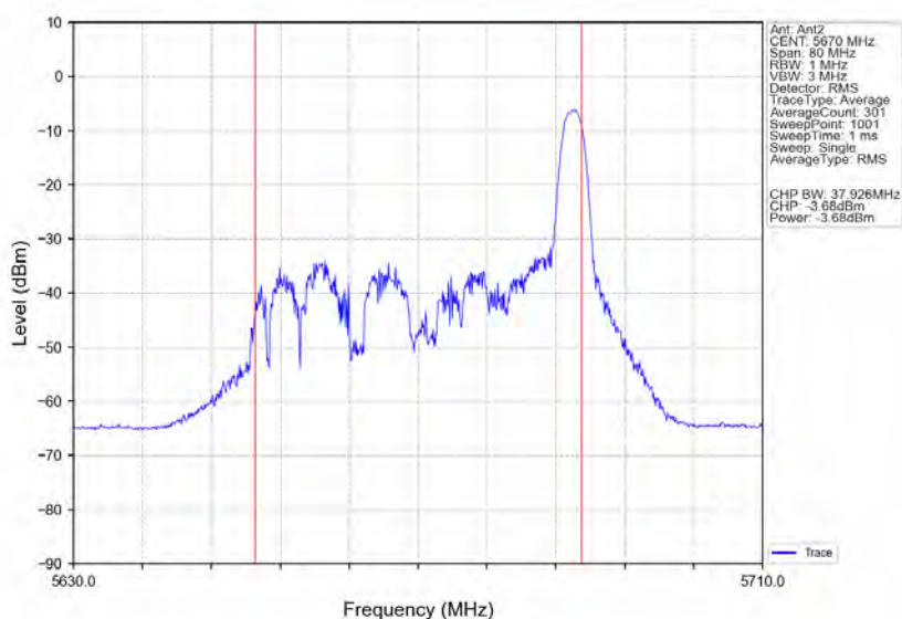
802.11ax(HE40) HCH 5670MHz RU26 Right Ant2 NTNv
