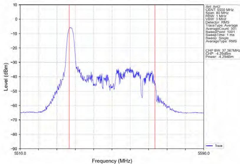
802.11ax(HE40) MCH_5550MHz RU26 Left Ant2 NTN
