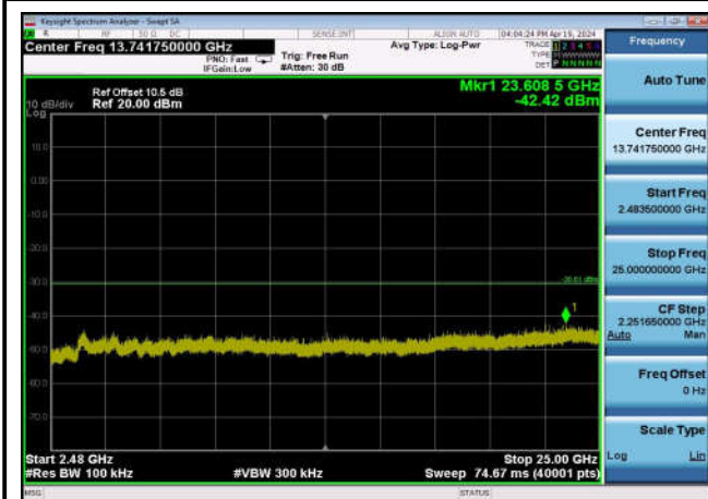
,Plot 4,2483.5MHz~25000MHz-802.11n(20 MHz),2437MHz,Ant0
