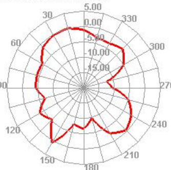
2400.000MHz E1
