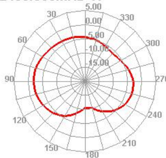
2400.000MHz H
