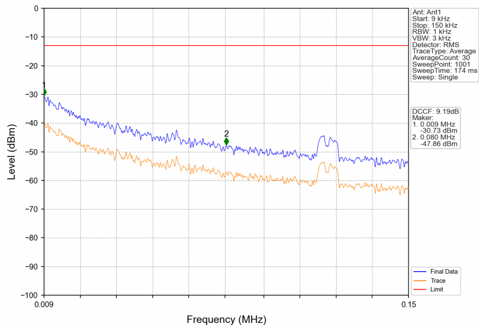
GSM850_EGPRS_HCH_848.8MHz_1 TX Slot_NTNV
