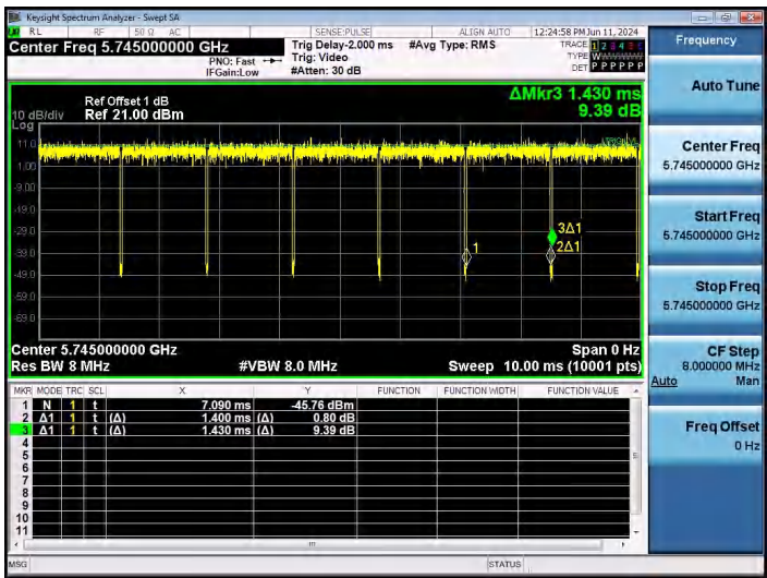
NTNV-11A-Ant1-5745
