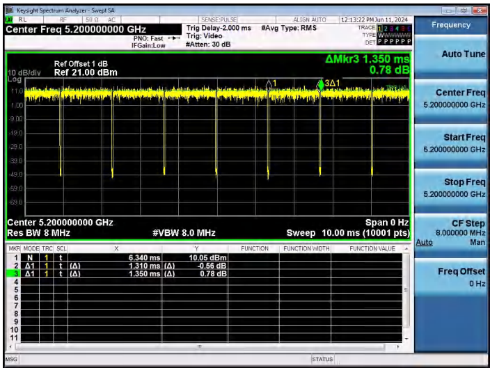
NTVN-11AC20SISO-Ant1-5200
