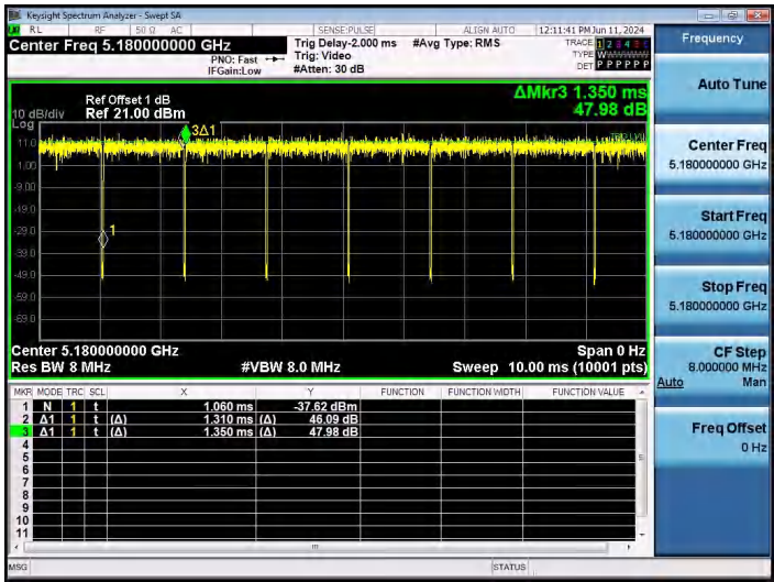
NTVN-11AC20SISO-Ant1-5180
