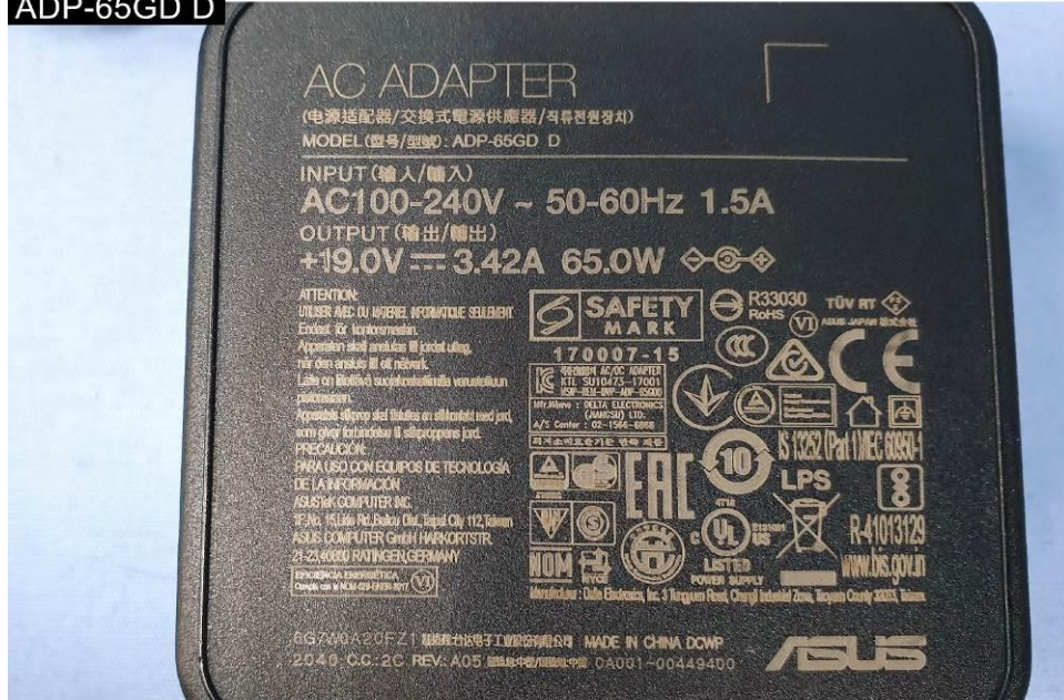
EUT Photo (24)
