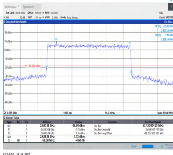
1-N41-30-70-H-9-CP-256QAM-Outer_Full-189@0-A nt1-67.42-69.580-≤70-PASS
