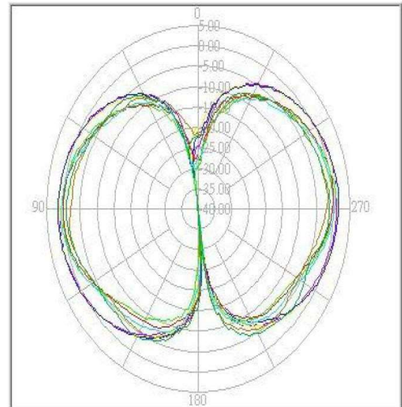
E-Plane
