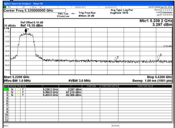
802.11 a 5240MHz
