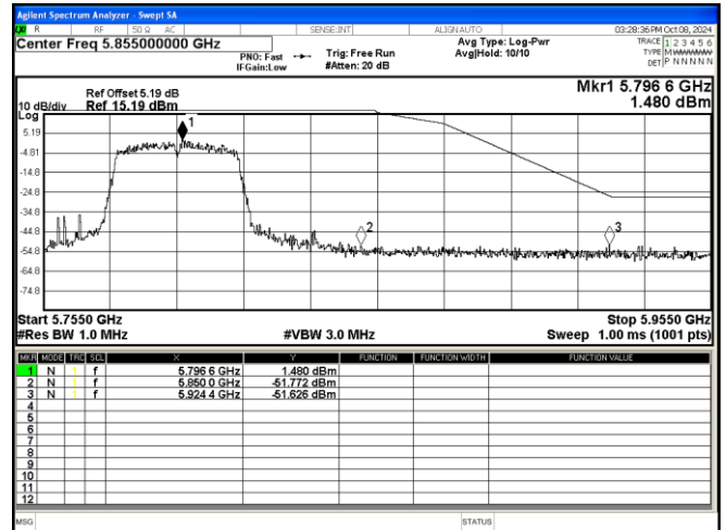
802.11 n40 5795MHz
