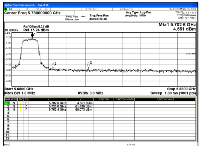
802.11 a 5700MHz
