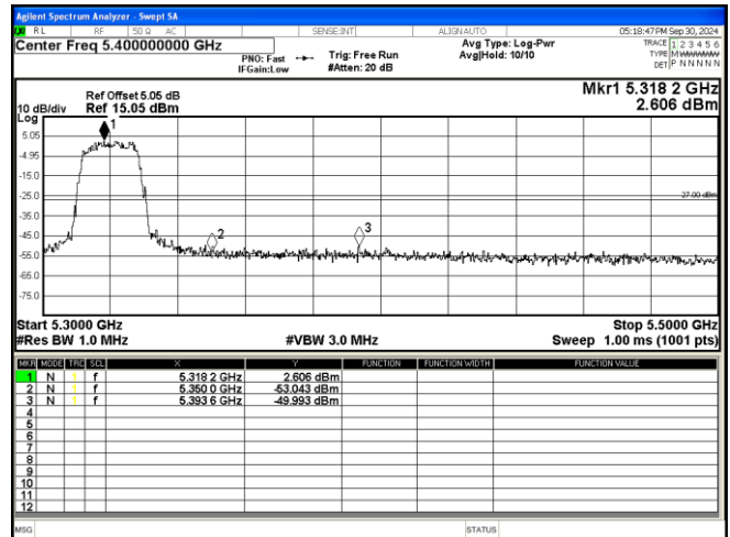
802.11 a 5320MHz
