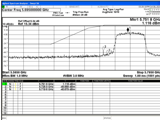
802.11 n40 5755MHz
