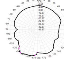
2500.0MHz Total(E2-YZ), Max: 3.13dB
