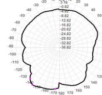
2490.0MHz Total(E2-YZ), Max: 2.94dB
