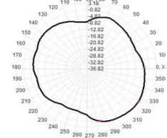
Total(H+V), Max: -1.75dB, Crd=11.32
