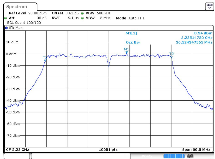
OBWac40 5230MHz Ant1
