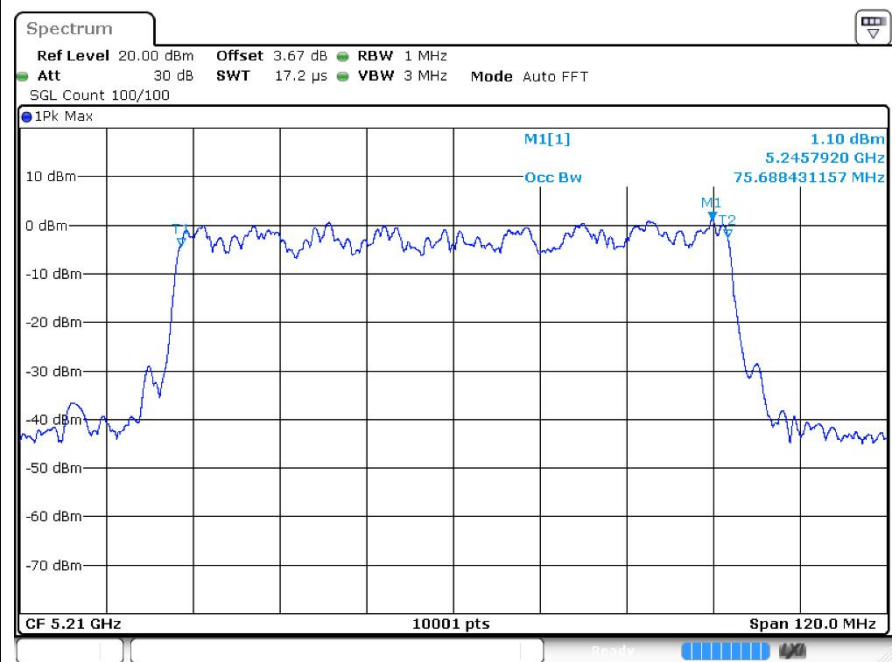
OBWac80 5210MHz Ant1
