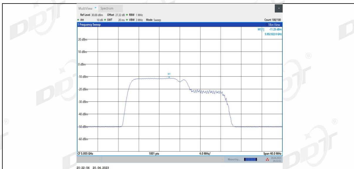
11BE20MIMO Ant4 5955 106+26 2
