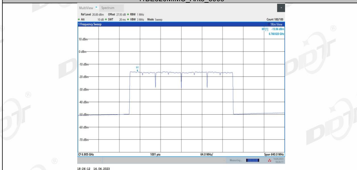
11BE320MIMO Ant4 6905
