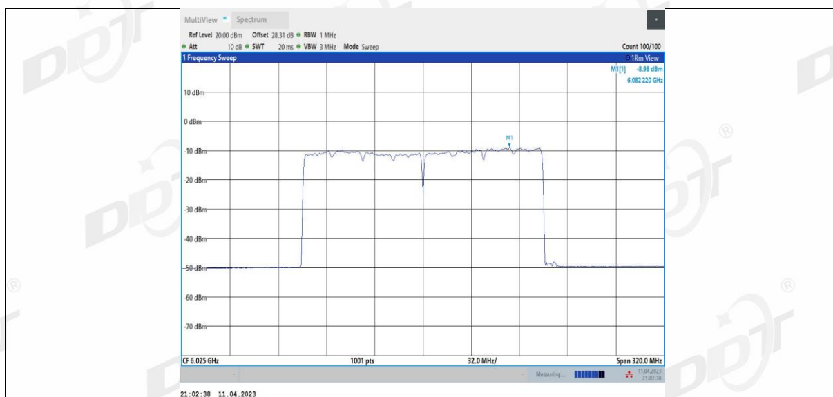
11BE160MIMO Ant4 6025
