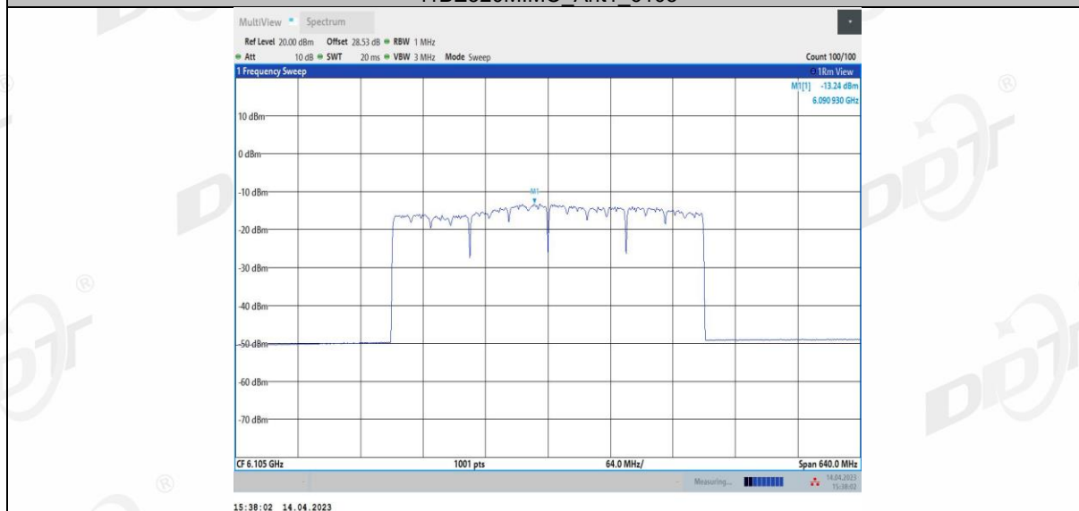
11BE320MIMO Ant2 6105
