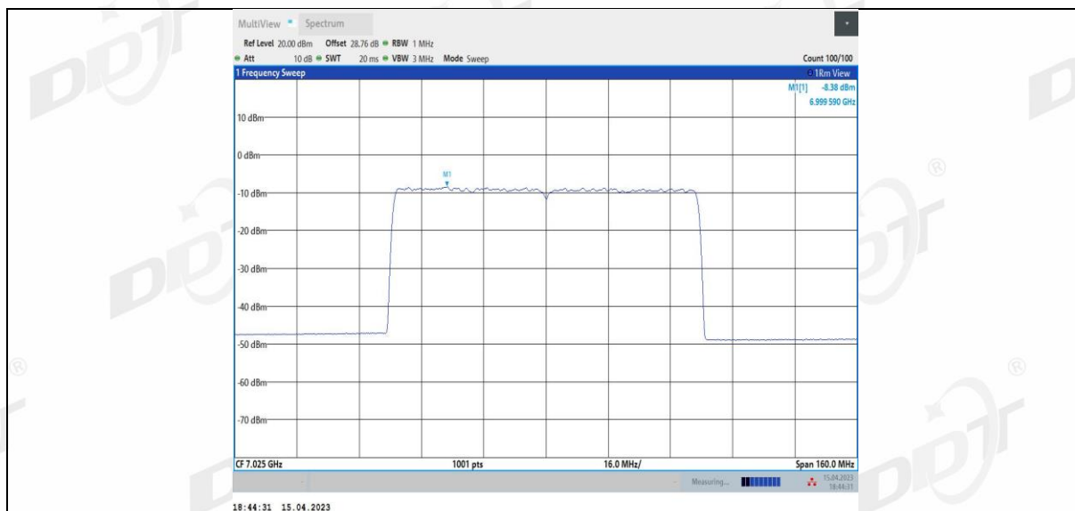
11BE80MIMO_Ant2_7025
