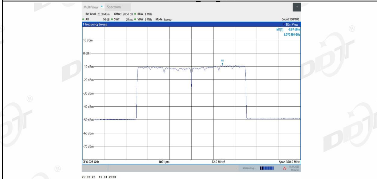
11BE160MIMO Ant3 6025
