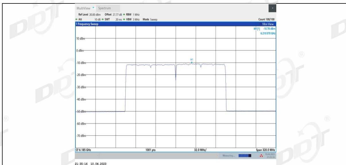
11BE160MIMO Ant3 6185
