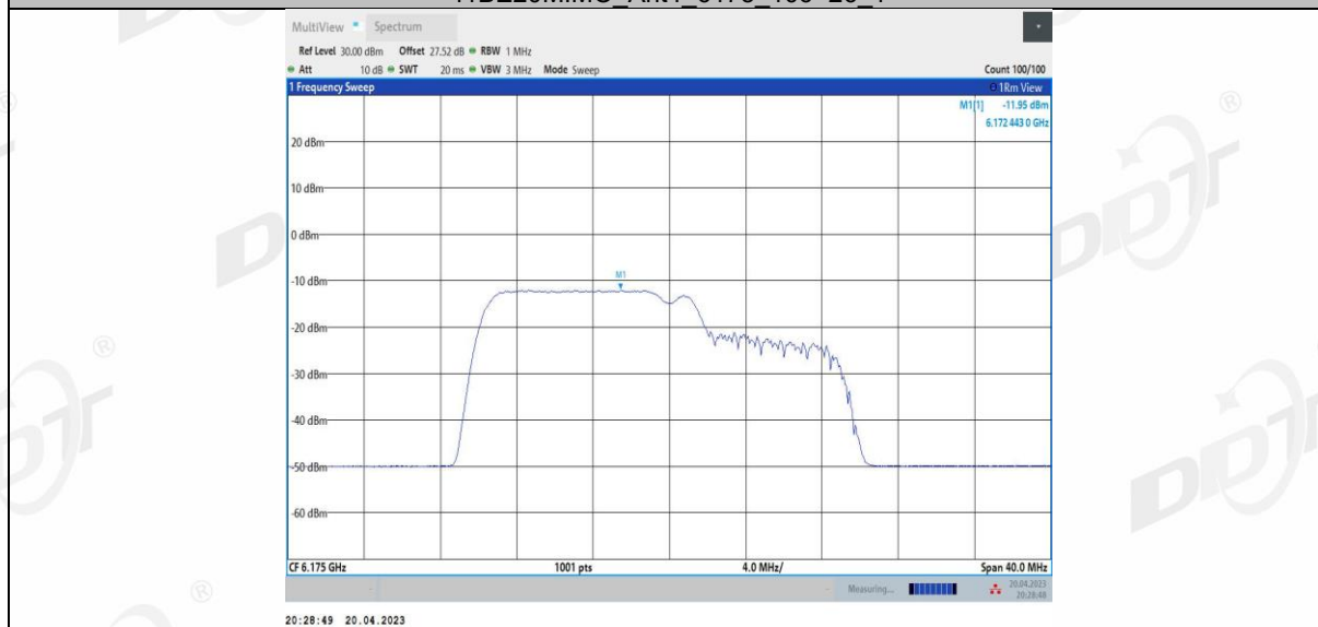
11BE20MIMO Ant4 6175 106+26 2
