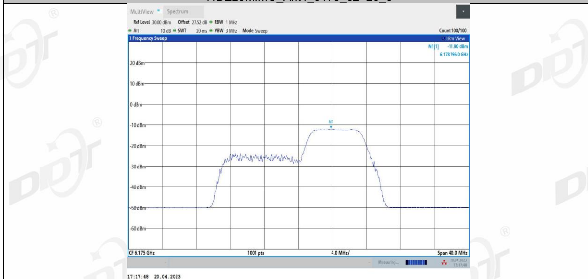
11BE20MIMO Ant4 6175 106+26 1
