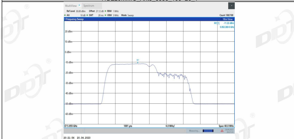
11BE20MIMO Ant3 5955 106+26 2
