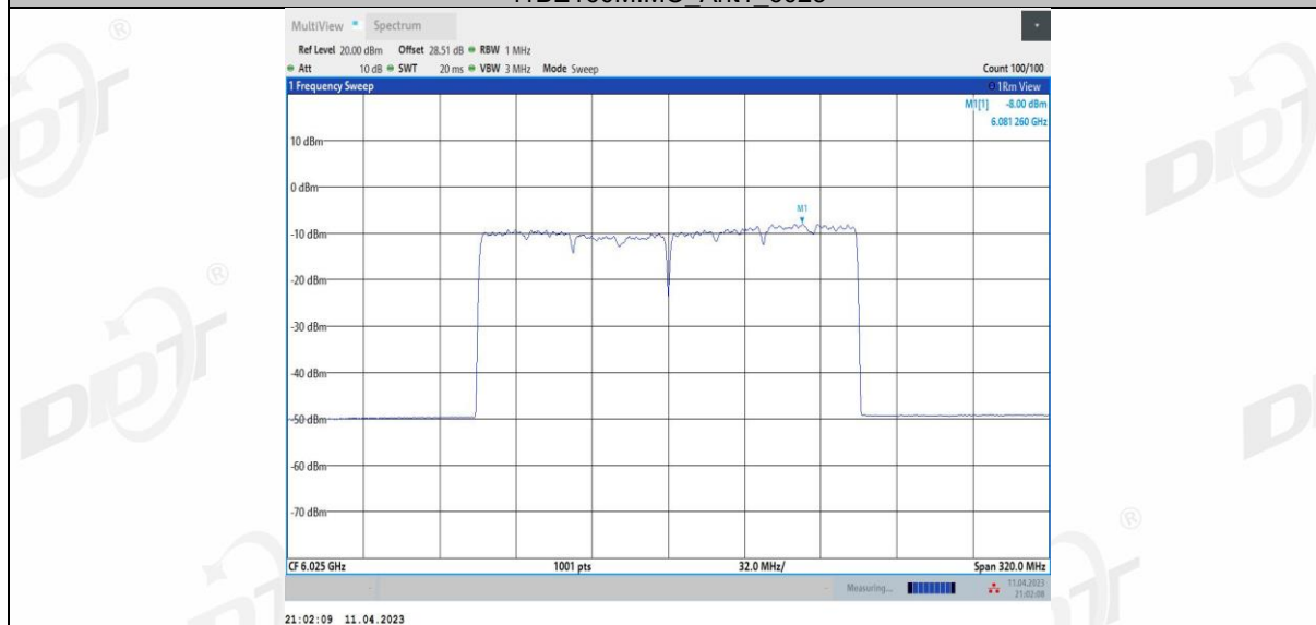
11BE160MIMO Ant2 6025
