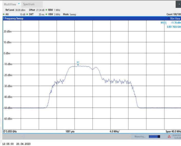
11BE20MIMO Ant1 5955 52+26 3
