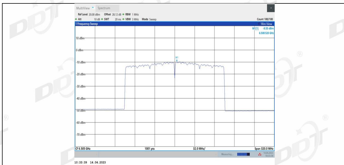
11BE160MIMO Ant4 6505
