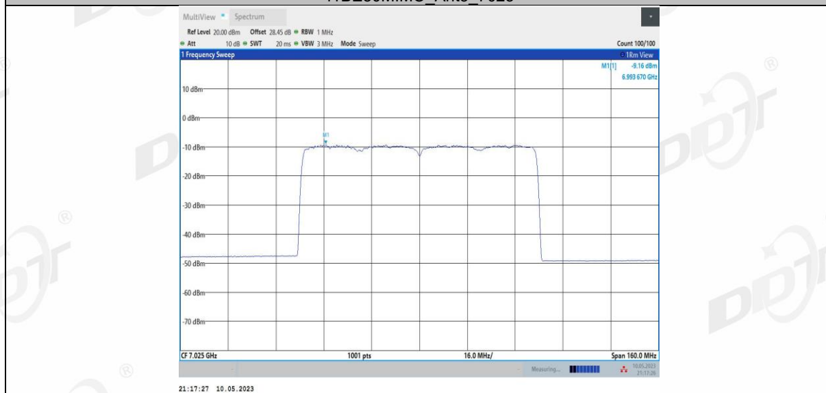
11BE80MIMO_Ant4_7025
