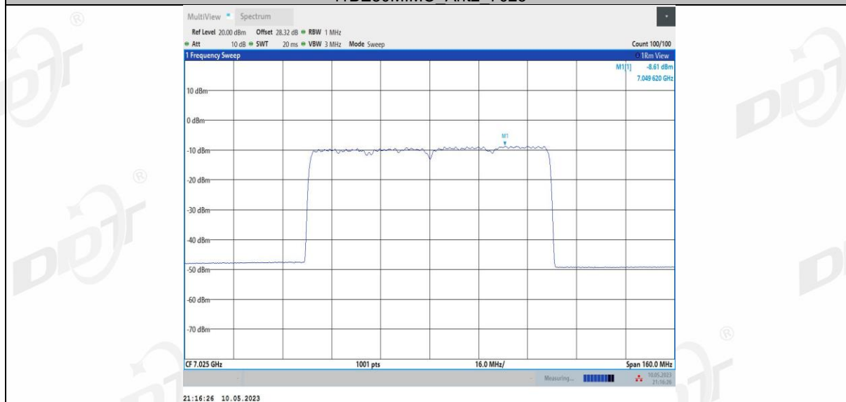
11BE80MIMO_Ant3_7025
