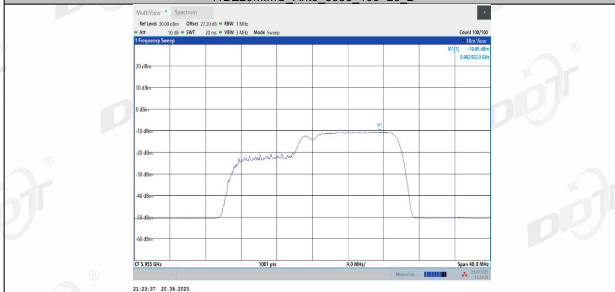
11BE20MIMO Ant4 5955 52+26 1
