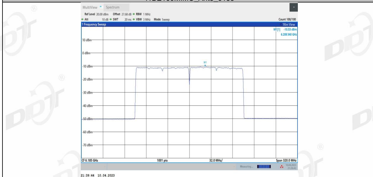
11BE160MIMO Ant4 6185
