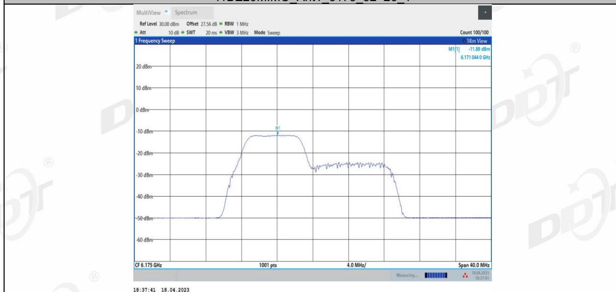
11BE20MIMO Ant1 6175 52+26 2
