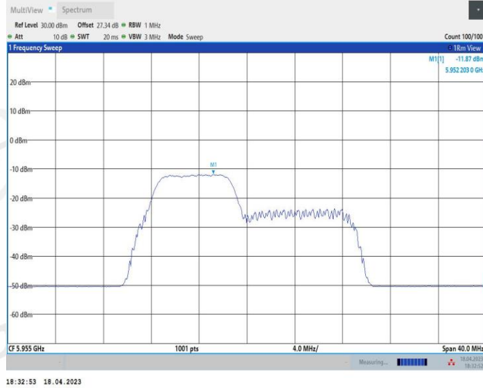
11BE20MIMO Ant1 5955 52+26 2
