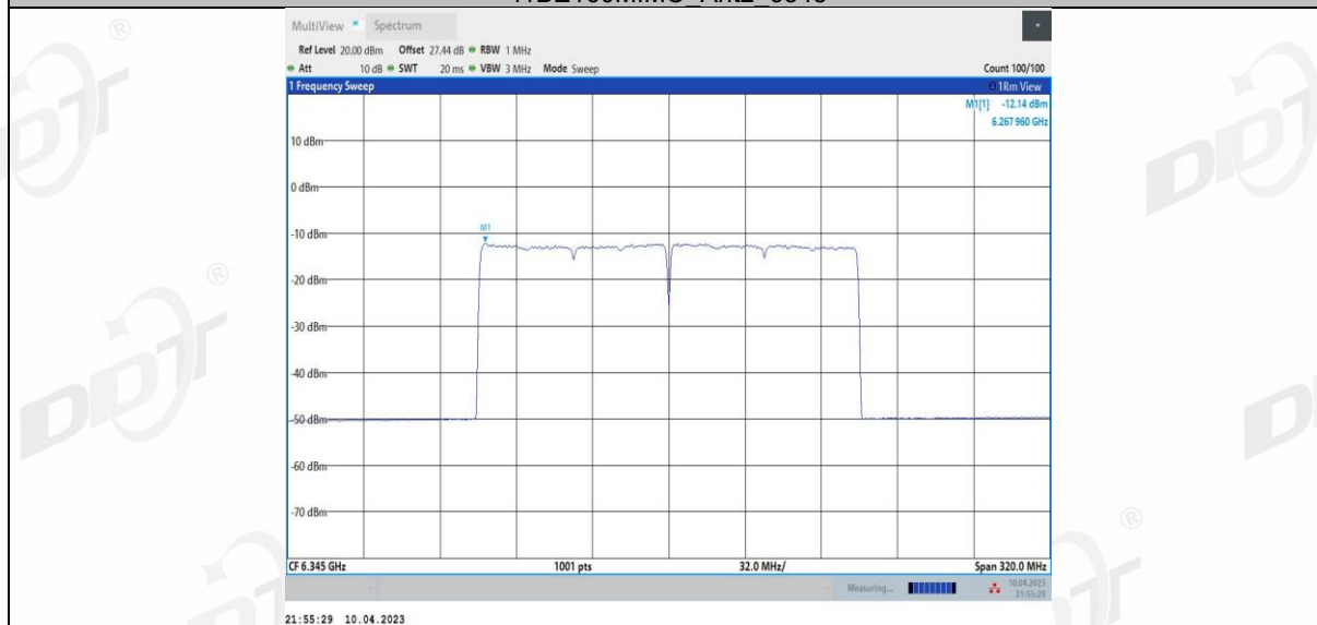
11BE160MIMO Ant3 6345
