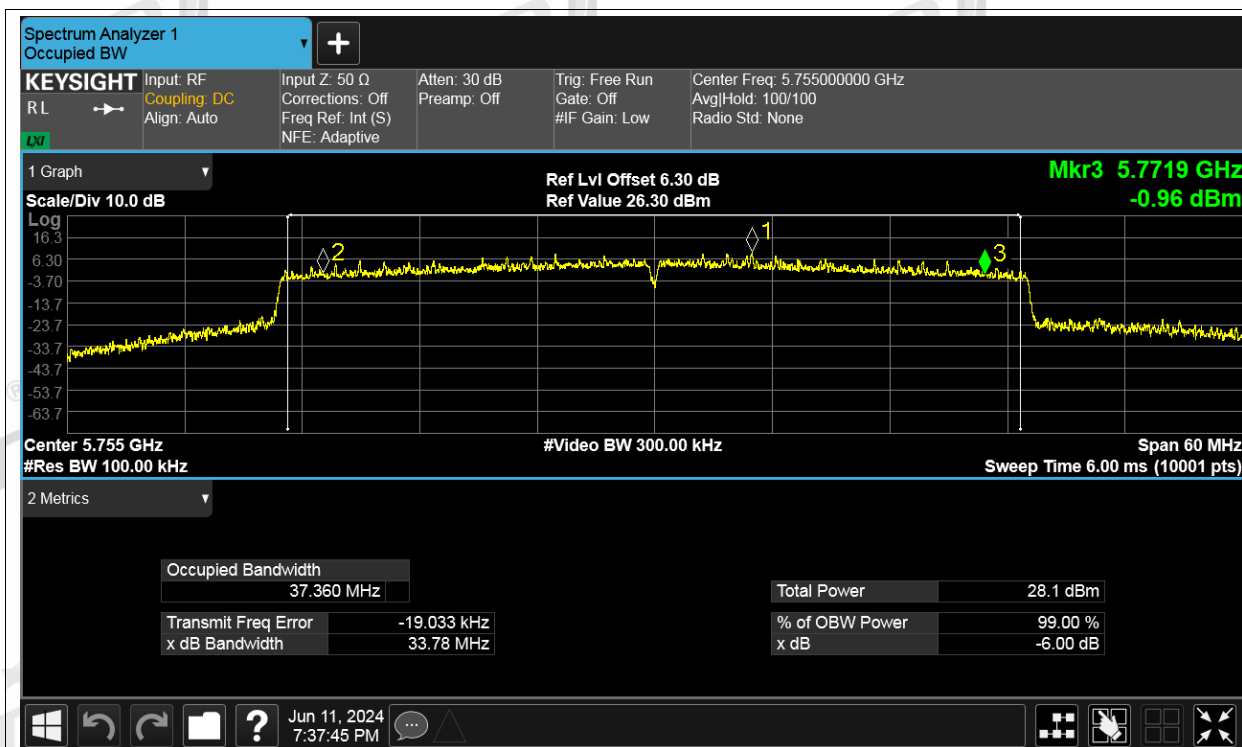
-6dB Bandwidth NVNT be40 5755MHz Ant2
