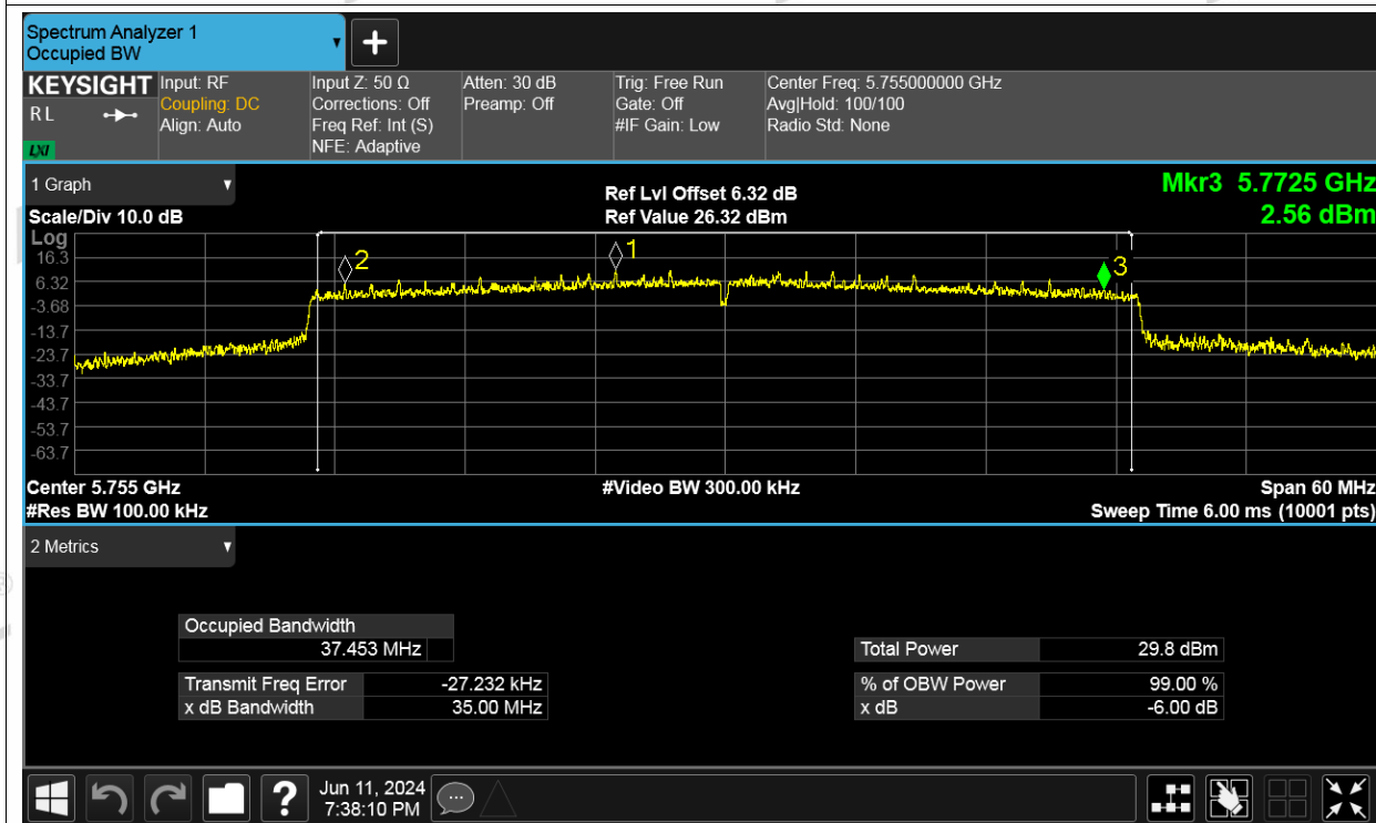
-6dB Bandwidth NVNT be40 5755MHz Ant3
