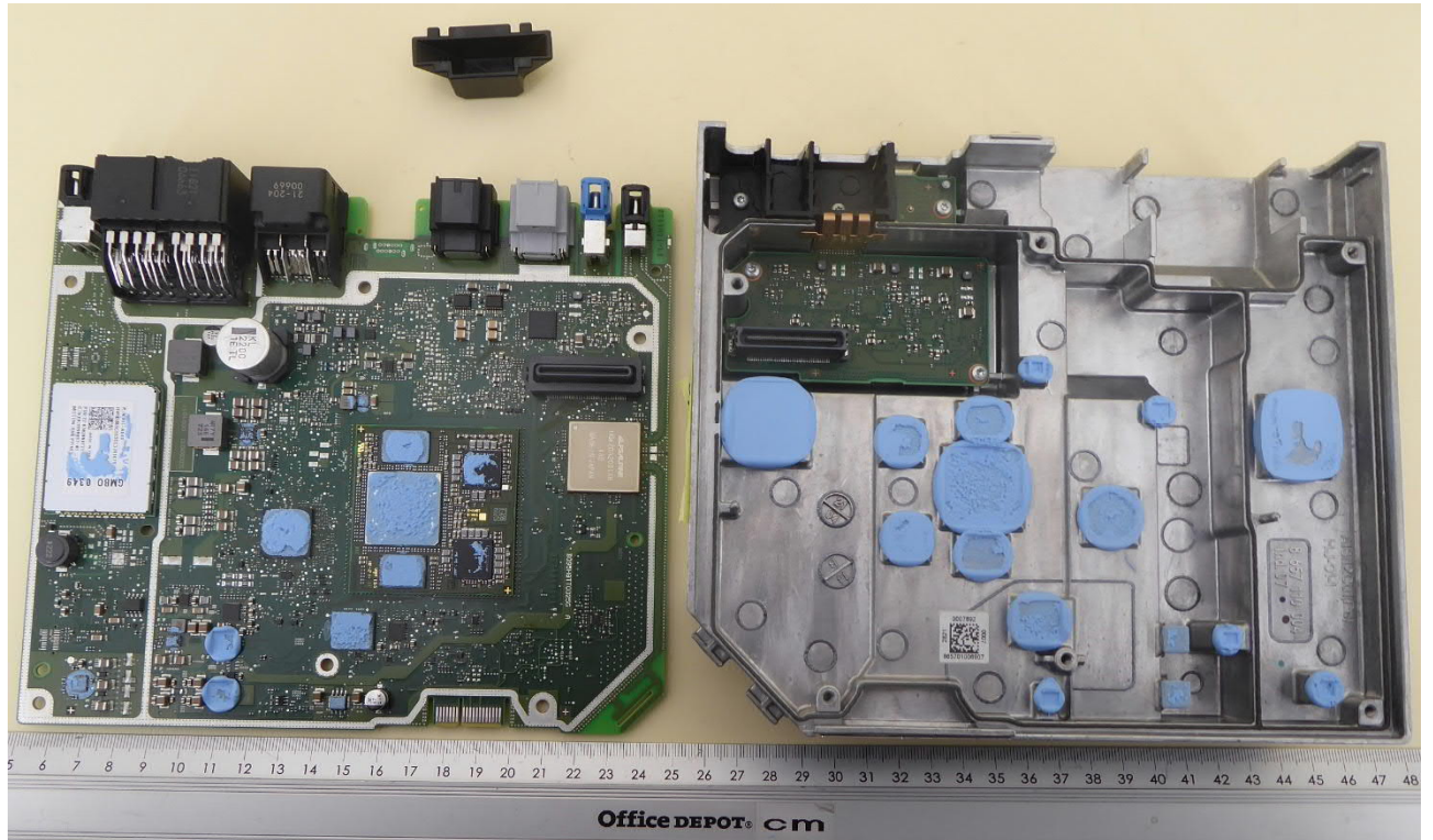
EUT open 2
