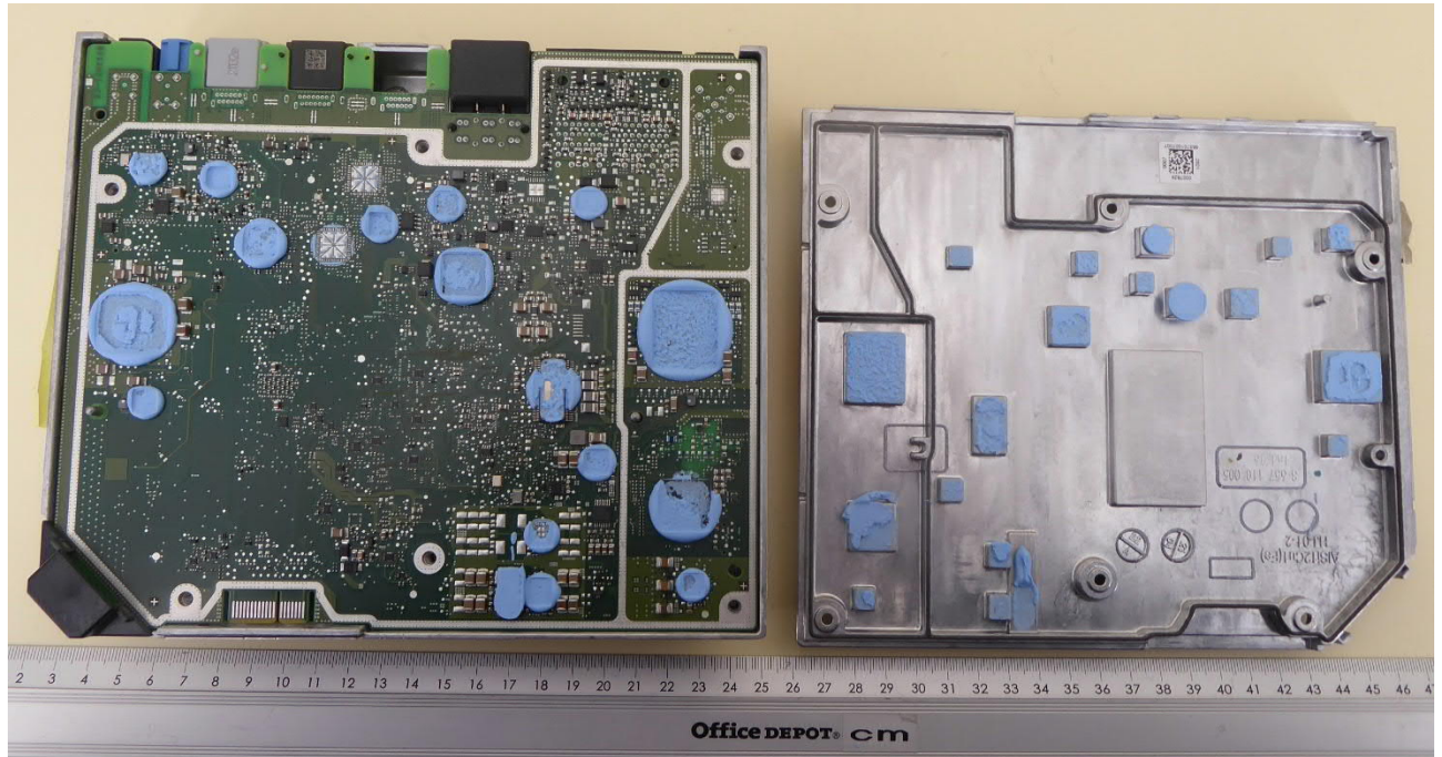
EUT open 1
