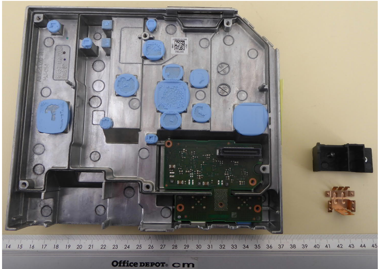
EUT open 4
