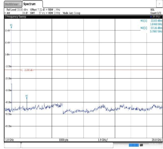
Band2-20MHz-QPSK-18700-1RB#0- Range2:1000~20000MHz
