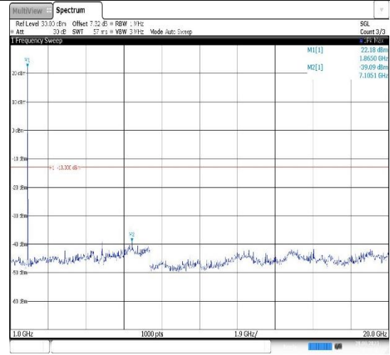
Band2-20MHz-QPSK-18900-1RB#0- Range2:1000~20000MHz
