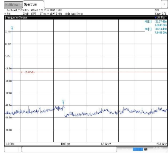
Band2-5MHz-QPSK-18900-1RB#0- Range2:1000~20000MHz
