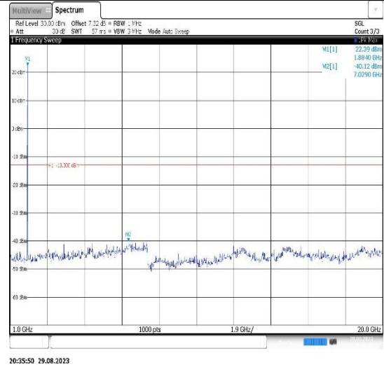
Band2-10MHz-QPSK-19150-1RB#0- Range2:1000~20000MHz
