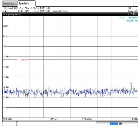
Band2-20MHz-QPSK-18700-1RB#0- Range1:30~1000MHz
