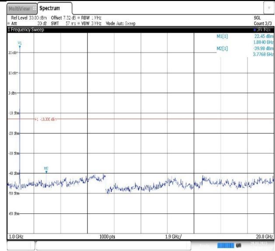
Band2-20MHz-16QAM-18700-1RB#0- Range2:1000~20000MHz
