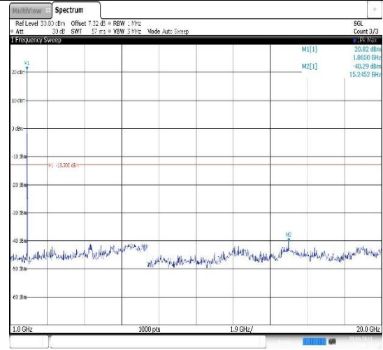
Band2-20MHz-16QAM-18900-1RB#0- Range2:1000~20000MHz
