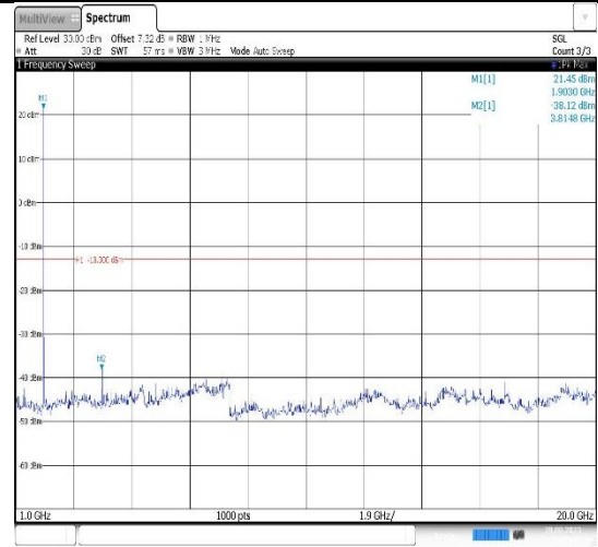
Band2-5MHz-QPSK-18625-1RB#0- Range2:1000~20000MHz
