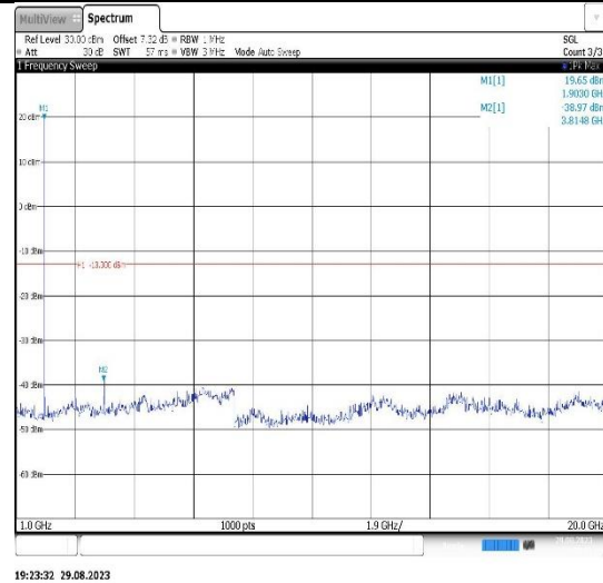
Band2-3MHz-QPSK-18615-1RB#0- Range2:1000~20000MHz
