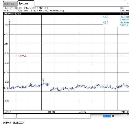
Band2-3MHz-QPSK-19185-1RB#0- Range2:1000~20000MHz
