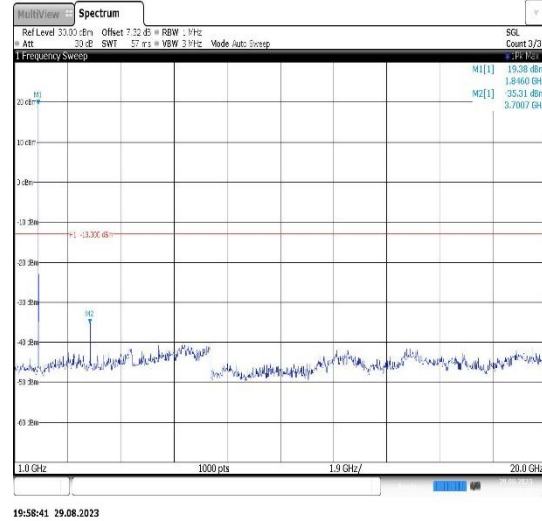
Band2-3MHz-QPSK-18900-1RB#0- Range2:1000~20000MHz
