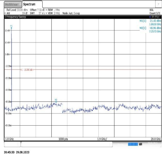
Band2-15MHz-QPSK-19125-1RB#0- Range2:1000~20000MHz
