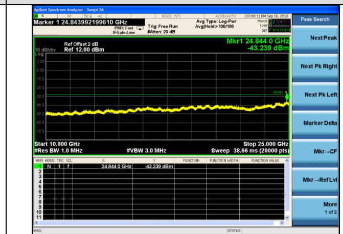
11nHT40-LCH
