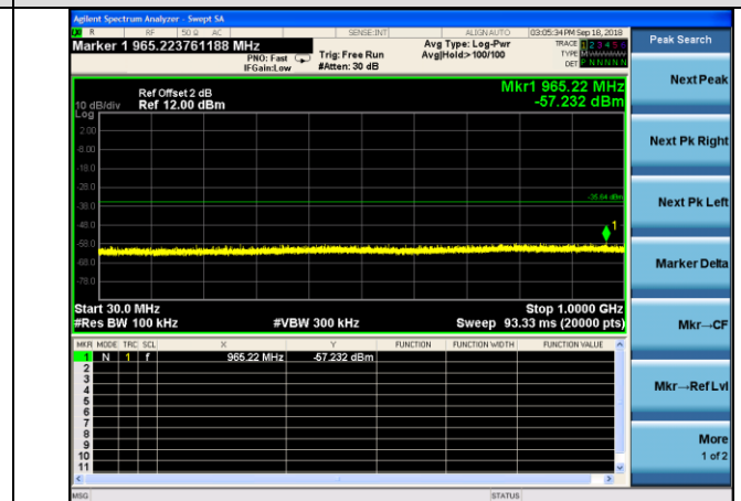
11nHT40-LCH
