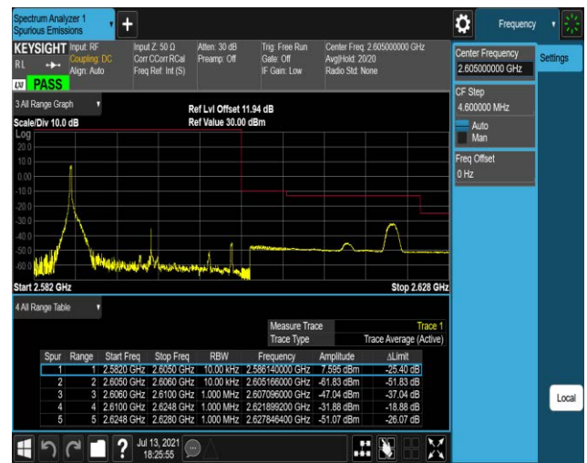
Band41-20MHz-QPSK-40640-100RB#0
