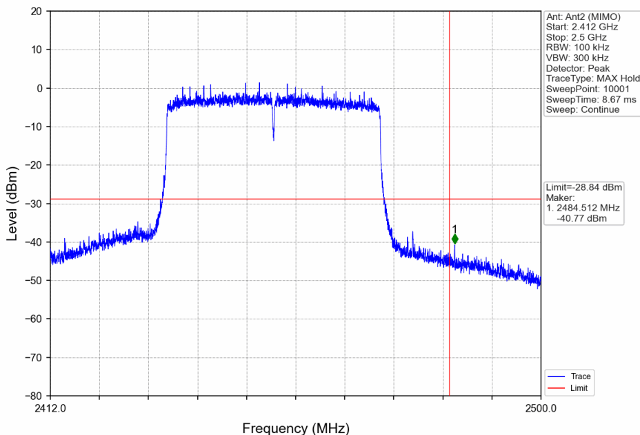
802.11ax(HEW40)_HCH_2452MHz_RU484_Left_Ant2 (MIMO)_NTNV
