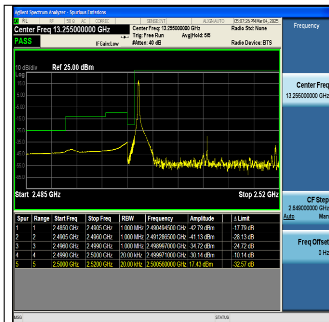
NTNV-n7-PC3-15-20-L-DFT-BPSK-Edge_1RB_Left-PASS
