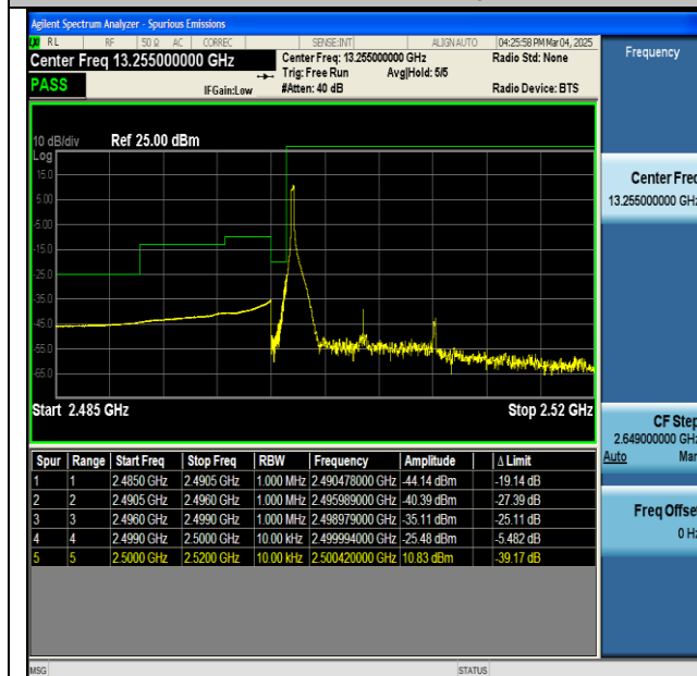
NTNV-n7-PC3-15-10-L-CP-QPSK-Edge_1RB_Left-PASS
