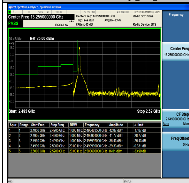
NTNV-n7-PC3-15-20-L-CP-QPSK-Edge_1RB_Left-PASS
