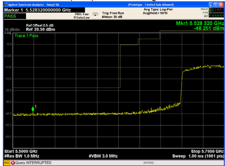
802.11ac(HT80) U-NII-3 Band edge-left side
