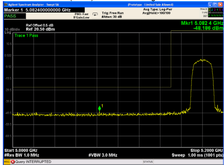
802.11ac(HT20) U-NII-1 Band edge-left side
