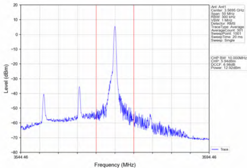
n78d 15kHz SISO NTNv 20MHz CP-OFDM QPSK 3560.01MHz Edge 1RB Right
