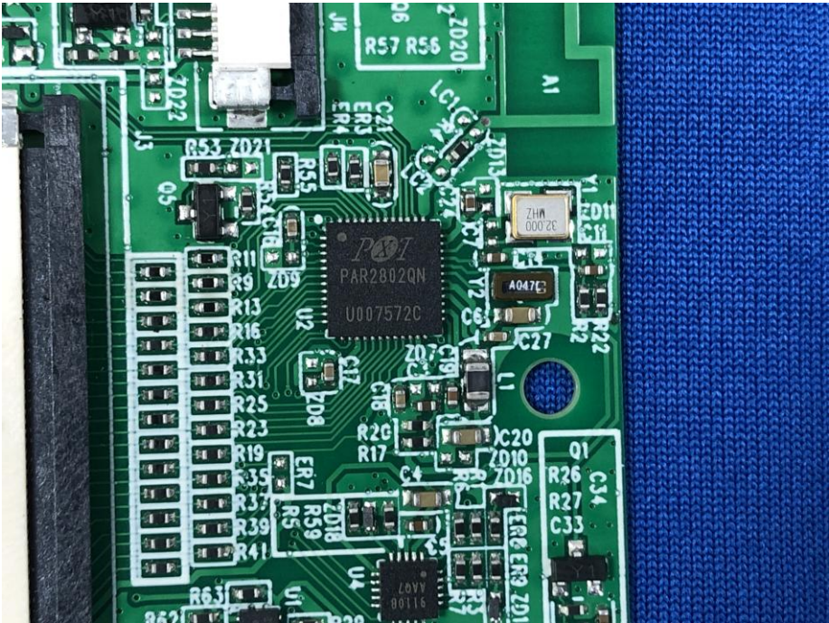
EUT Photo 19
