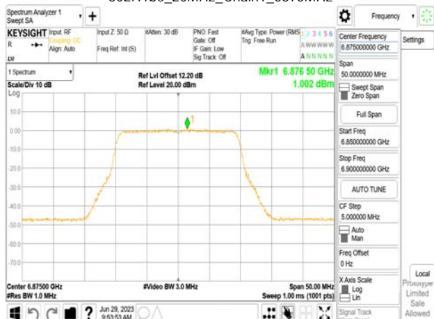
802.11be_20MHz_Chain1_6875MHz
