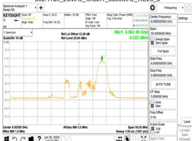
802.11be_20MHz_Chain1_6855MHz_RU52_40
