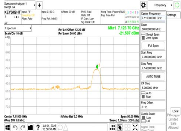
802.11be_20MHz_Chain0_7115MHz_RU52_40
