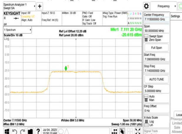
802.11be_20MHz_Chain0_7115MHz
