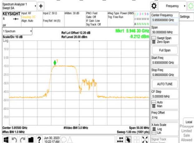
802.11be_20MHz_Chain1_5955MHz_RU106_53
