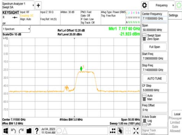
802.11be_20MHz_Chain1_7115MHz_RU106_54
