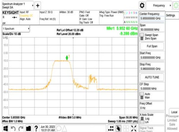
802.11be_20MHz_Chain1_5955MHz_RU106_53
