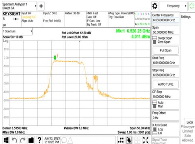
802.11be_20MHz_Chain1_6535MHz_106+26_MR1
