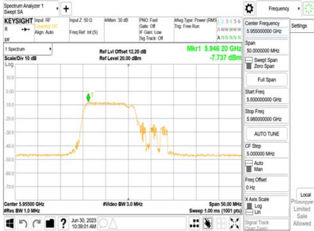
802.11be_20MHz_Chain0_5955MHz_52+26_MRU1
