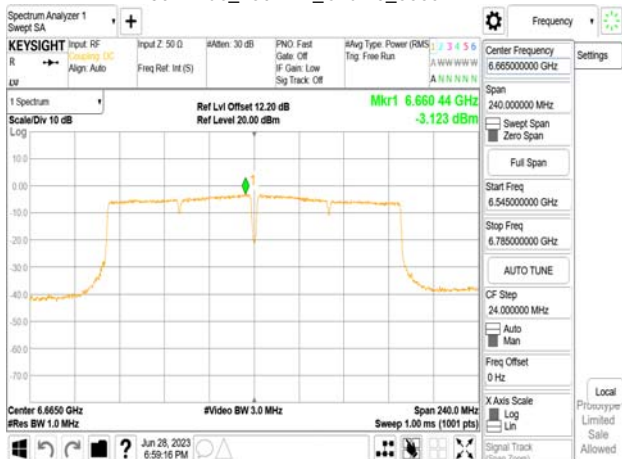
802.11ac_160MHz_Chain0_6665MHz
