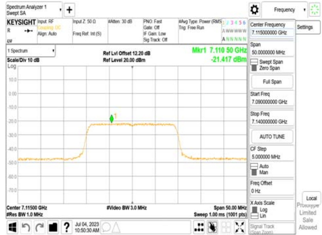
802.11be_20MHz_Chain1_7115MHz_106+26_MR2
