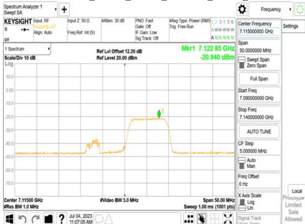
802.11be_20MHz_Chain0_7115MHz_RU106_54
