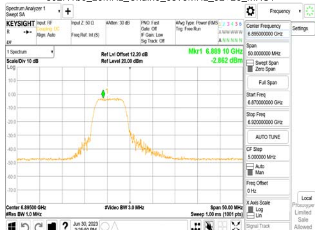
802.11be_20MHz_Chain0_6895MHz_RU106_53
