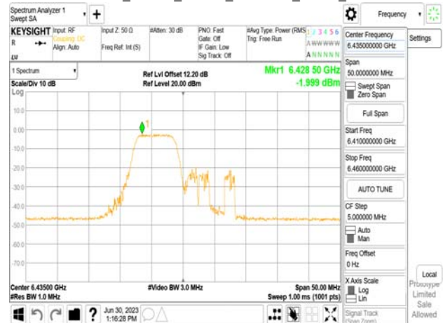
802.11be_20MHz_Chain0_6435MHz_RU106_53
