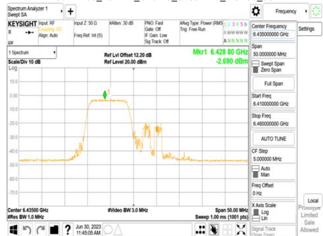
802.11be_20MHz_Chain0_6435MHz_RU26_0
