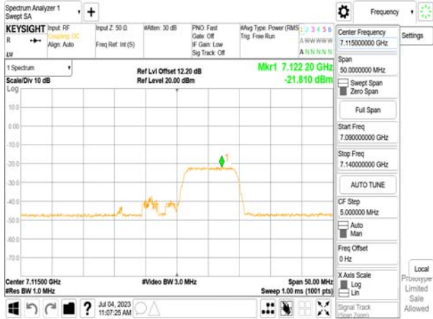
802.11be_20MHz_Chain1_7115MHz_RU26_8
