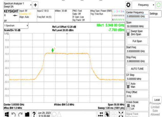
802.11be_20MHz_Chain1_5955MHz
