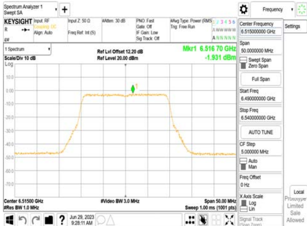
802.11be_20MHz_Chain1_6515MHz_106+26_MRUI2
