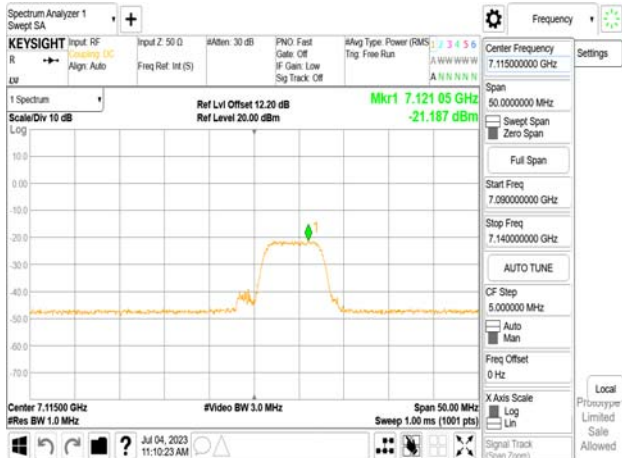
802.11be_20MHz_Chain0_7115MHz_RU106_54
