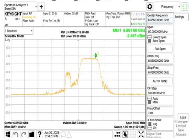
802.11be_20MHz_Chain1_6855MHz_RU106_54
