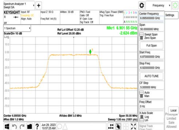
802.11be_20MHz_Chain0_6895MHz_106+26_MRUI
