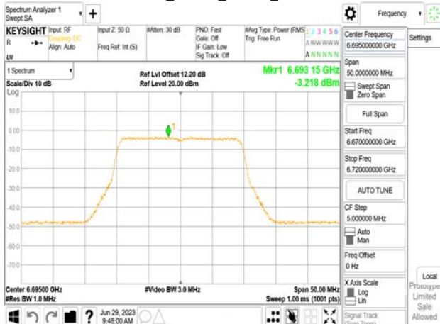
802.11be_20MHz_Chain0_6695MHz
