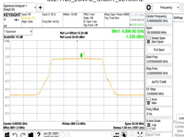
802.11be_20MHz_Chain1_6895MHz_106+26_MRU1
