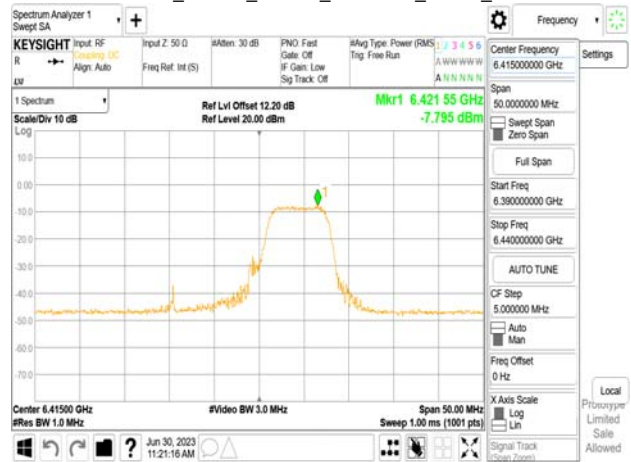
802.11be_20MHz_Chain0_6415MHz_RU106_54
