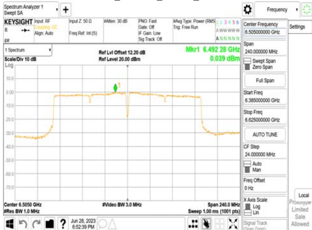
802.11ac_160MHz_Chain1_6505MHz
