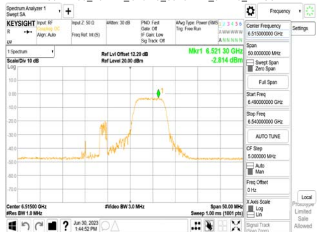
802.11be_20MHz_Chain0_6515MHz_RU106_54
