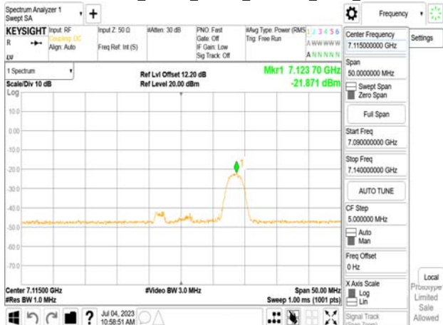
802.11be_20MHz_Chain1_7115MHz_RU26_8
