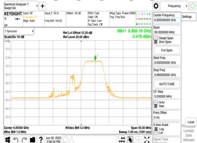
802.11be_20MHz_Chain0_6855MHz_52+26_MRU3
