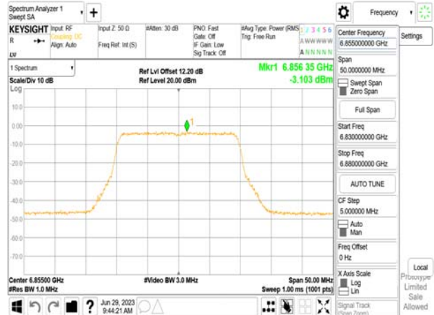
802.11be_20MHz_Chain0_6855MHz_106+26_MRU2
