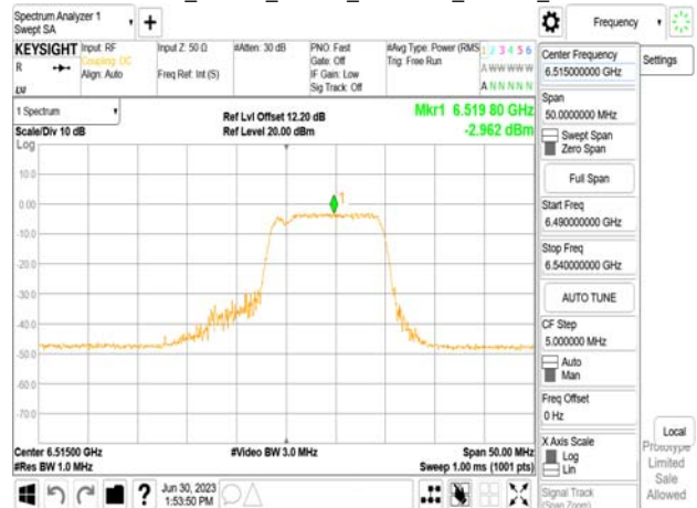
802.11be_20MHz_Chain0_6515MHz_52+26_MRU3
