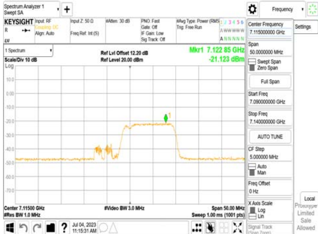
802.11be_20MHz_Chain0_7115MHz_52+26_MRU3
