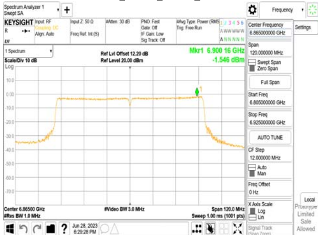
802.11ac_80MHz_Chain0_6865MHz
