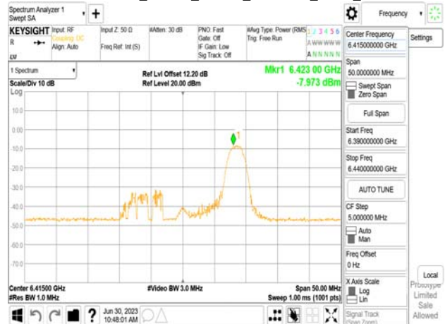
802.11be_20MHz_Chain0_6415MHz_RU26_8
