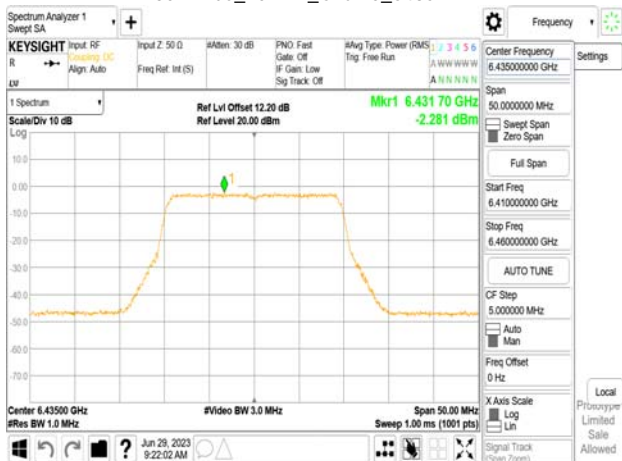
802.11be_20MHz_Chain0_6435MHz_106+26_MRUI
