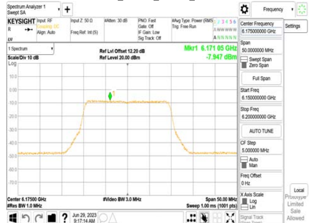
802.11be_20MHz_Chain1_6175MHz
