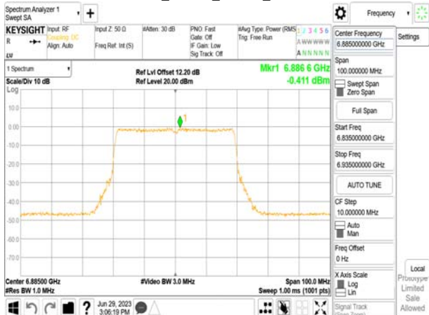
802.11be_40MHz_Chain1_6885MHz
