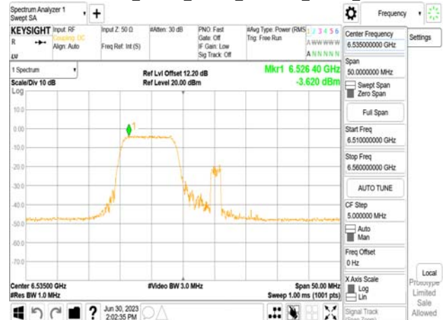
802.11be_20MHz_Chain0_6535MHz_RU106_53
