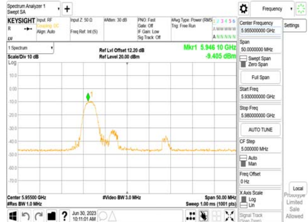
802.11be_20MHz_Chain1_5955MHz_RU52_37
