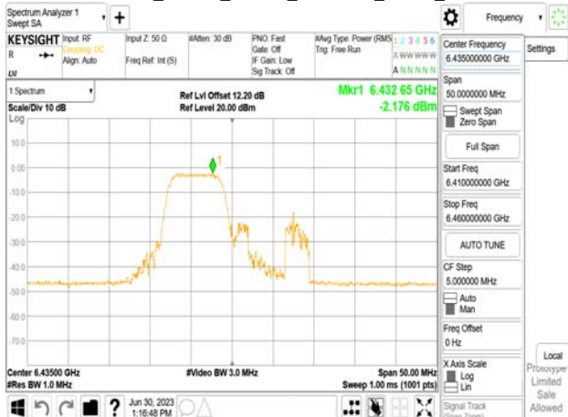
802.11be_20MHz_Chain1_6435MHz_52+26_MRU1
