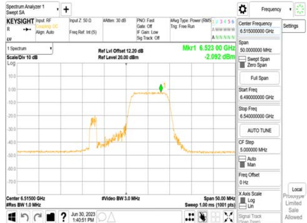
802.11be_20MHz_Chain1_6515MHz_RU26_8
