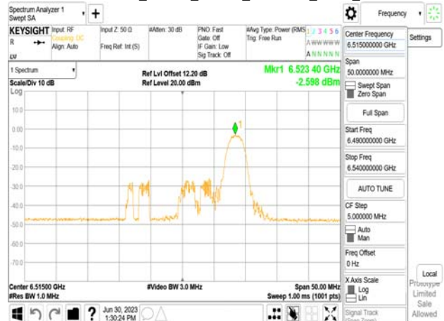
802.11be_20MHz_Chain1_6515MHz_RU26_8
