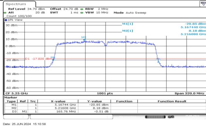
11AC160MIMO_Ant1_5250
