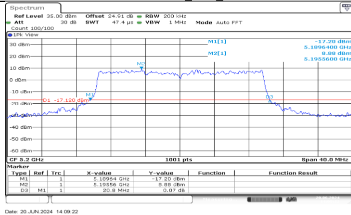
11AX20MIMO_Ant4_5200
