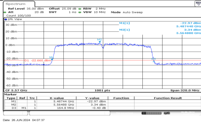
11AC160MIMO_Ant3_5570
