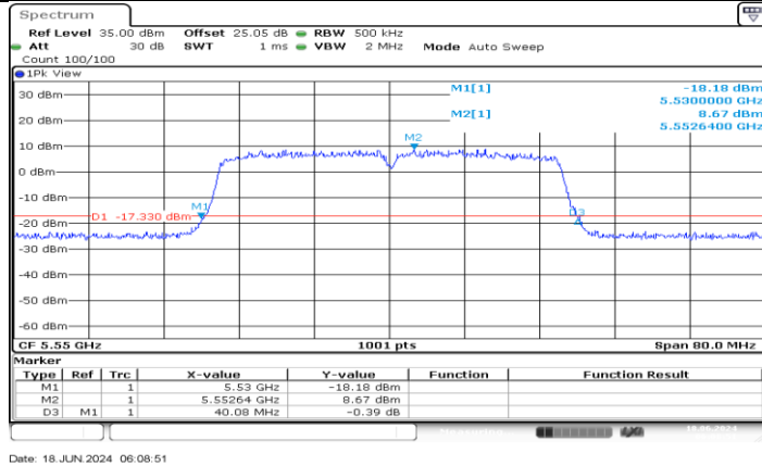
11AC40MIMO_Ant4_5550
