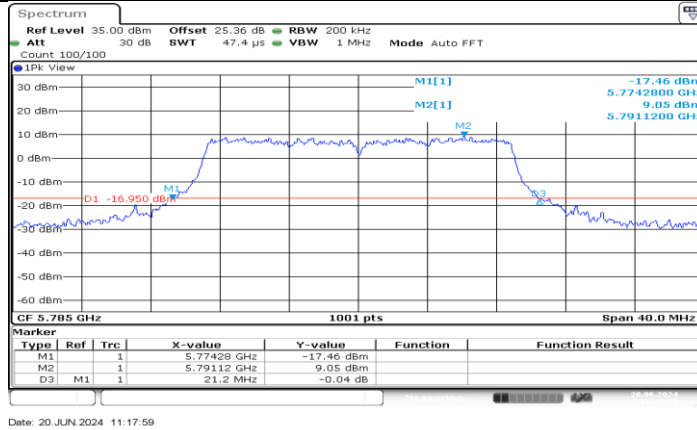
11AC20MIMO_Ant3_5785
