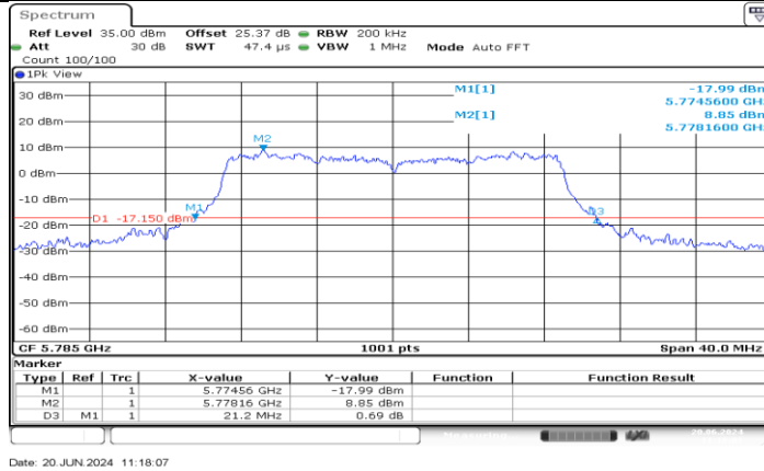
11AC20MIMO_Ant4_5785
