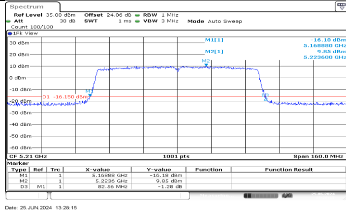
11AC80MIMO_Ant3_5210
