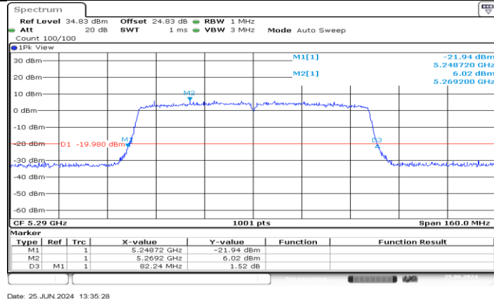
11AC80MIMO_Ant2_5290
