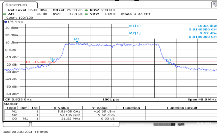
11AC20MIMO_Ant1_5825
