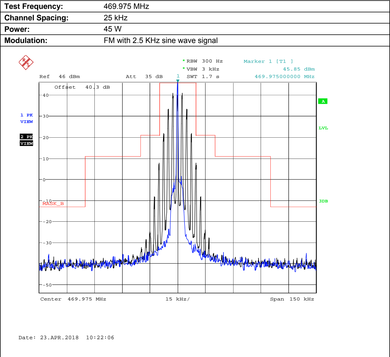
Plot 5.8.4.3.5. Emission Mask B, High Power
