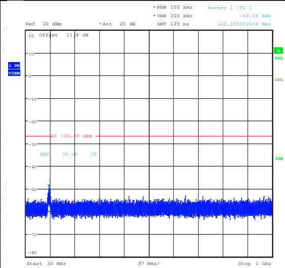
11G-Ant1-2437-30~1000-PASS
