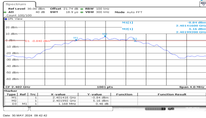
BLE_2M_Ant1_2402
