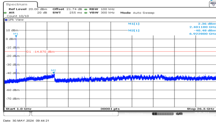
BLE_2M_Ant1_2402_1000~26500
