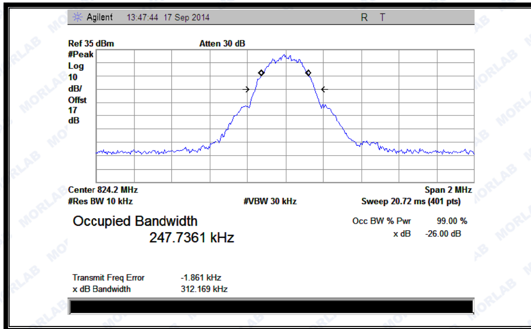
(Plot E1: GSM 850MHz Channel = 128)
