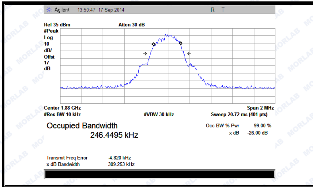
(Plot I1: GSM 1900MHz Channel = 661)
