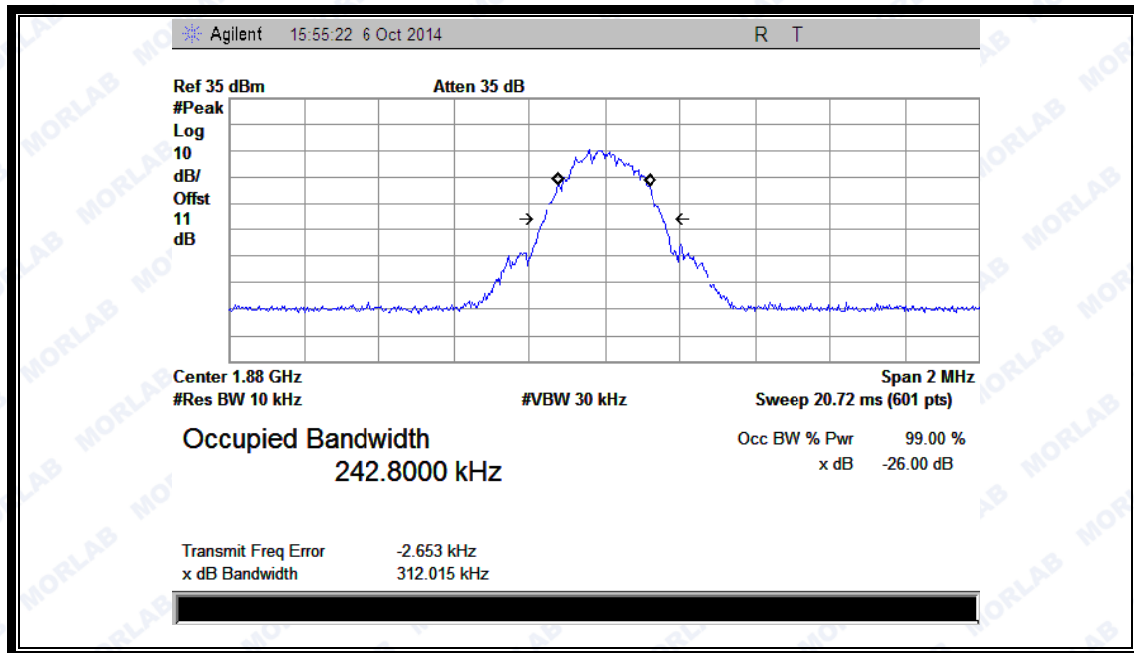
(Plot O1: GPRS 1900MHz Channel = 661)
