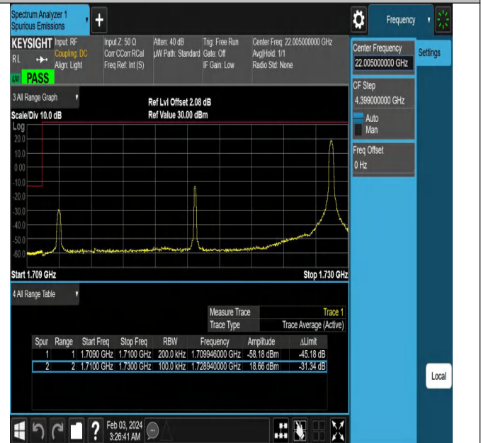
Band66_20MHz_QPSK_132072_1RB#99
