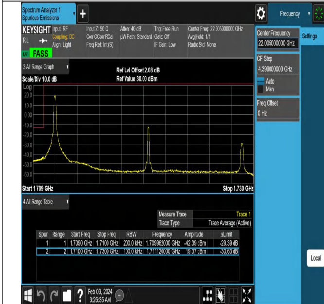
Band66_20MHz_QPSK_132072_1RB#0
