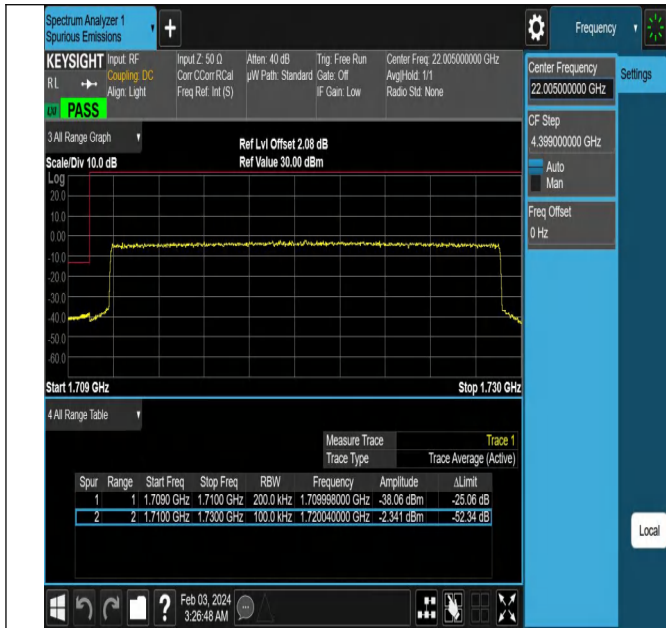
Band66_20MHz_QPSK_132072_100RB#0
