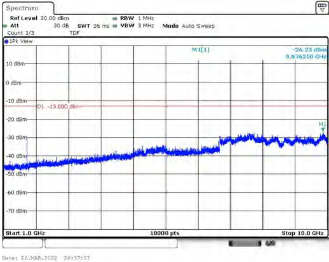
Band26-1.4MHz-QPSK-26797-1RB#0-Range2:1000~10000MHz
