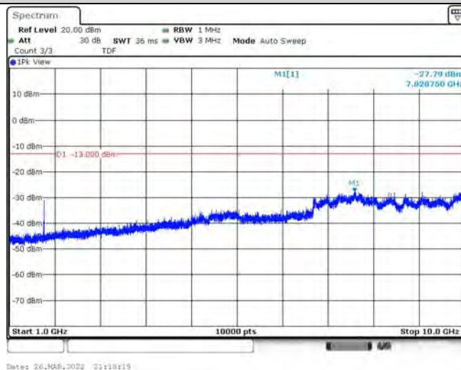
Band26-10MHz-QPSK-26990-1RB#0-Range2:1000~10000MHz
