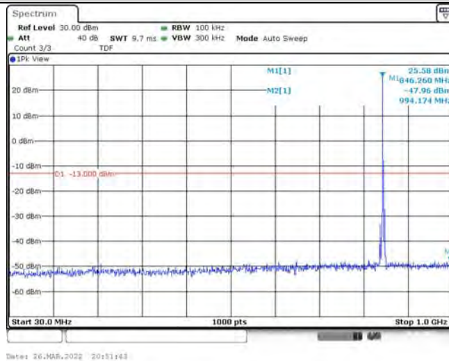
Band26-3MHz-QPSK-27025-1RB#0-Range1:30~1000MHz
