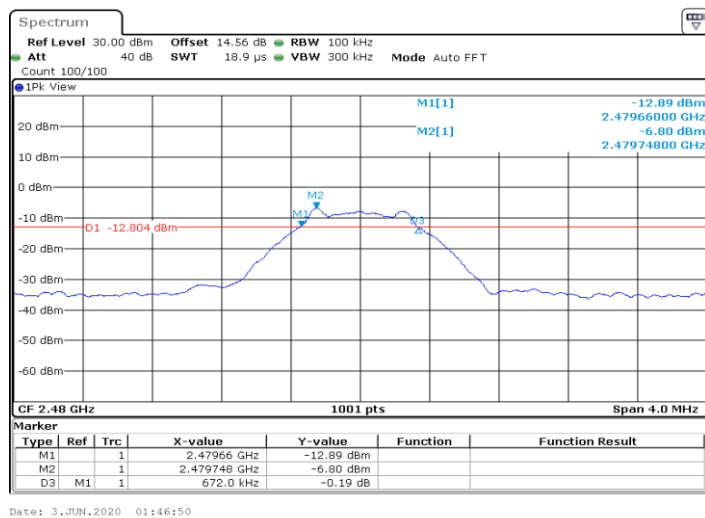
BLE_BT4.0_Ant1_2480
