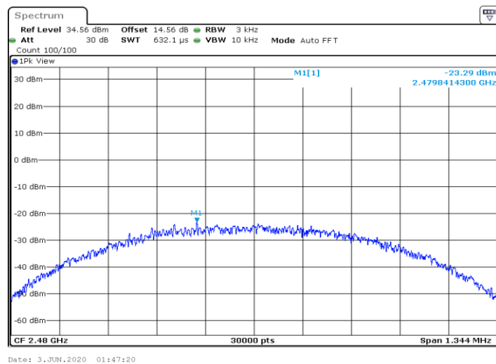
BLE_BT4.0_Ant1_2480
