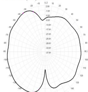
2440.0MHz Total(E1-XZ), Max= 2.09dBi
