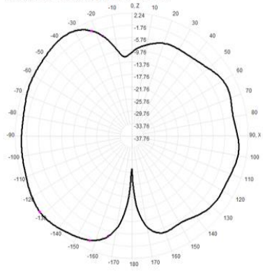
2480.0MHz Total(E1-XZ), Max= 2.24dBi
