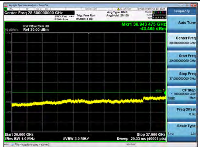
Band48-20G-37G / 15MHz / Low CH / 16QAM
