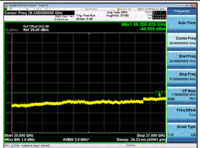
Band48-20G-37G / 20MHz / High CH / 16QAM
