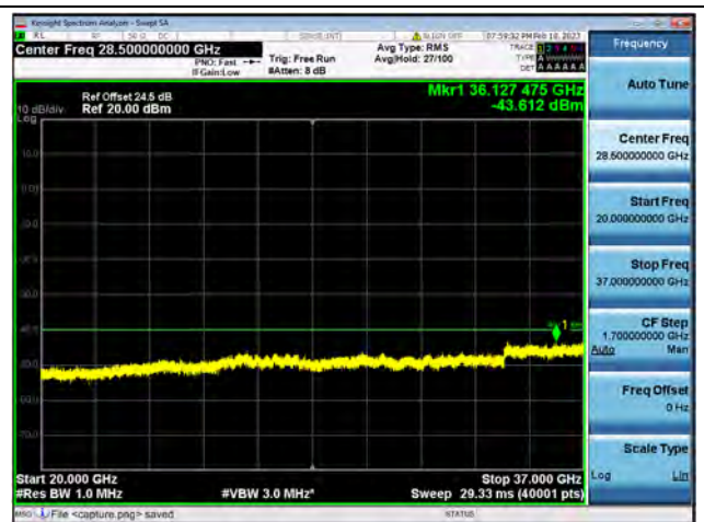
Band48-20G-37G / 20MHz / Mid CH / QPSK
