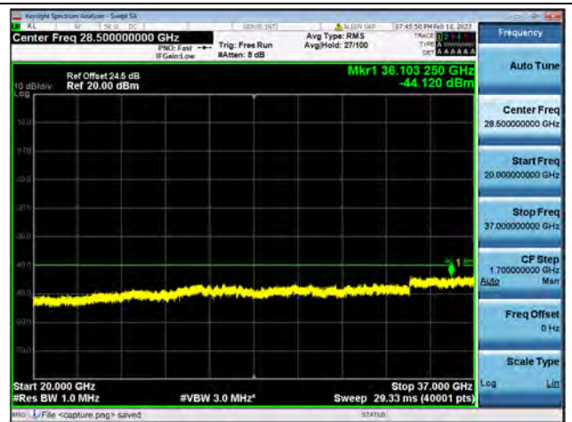
Band48-20G-37G / 10MHz / Low CH / 64QAM
