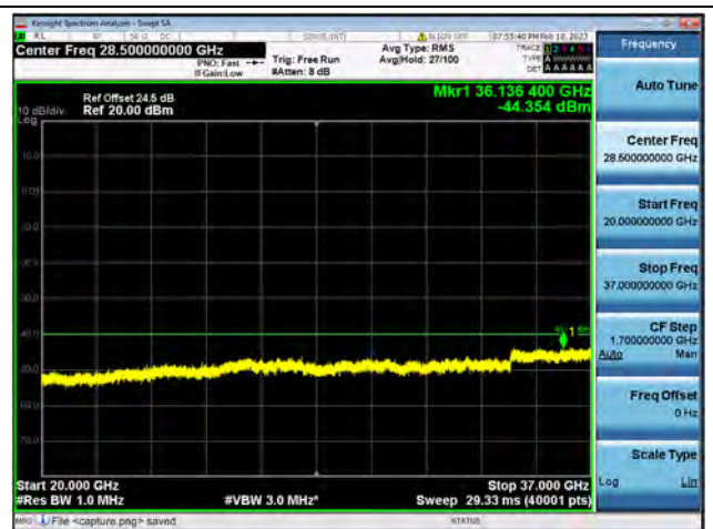
Band48-20G-37G / 15MHz / Mid CH / QPSK
