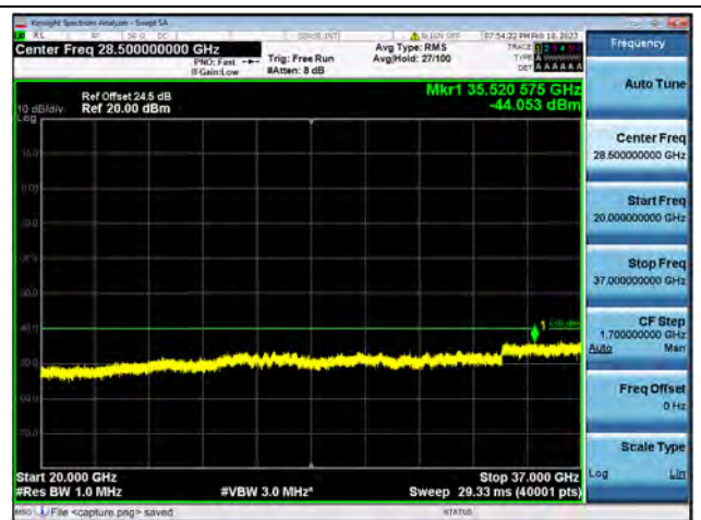
Band48-20G-37G / 15MHz / Low CH / QPSK
