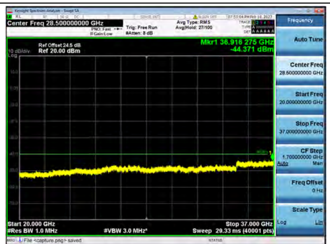
Band48-20G-37G / 10MHz / High CH / QPSK
