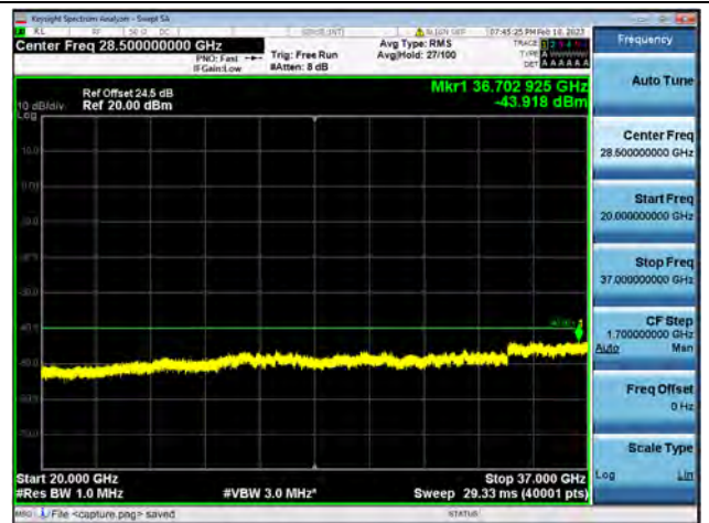
Band48-20G-37G / 10MHz / Low CH / 16QAM
