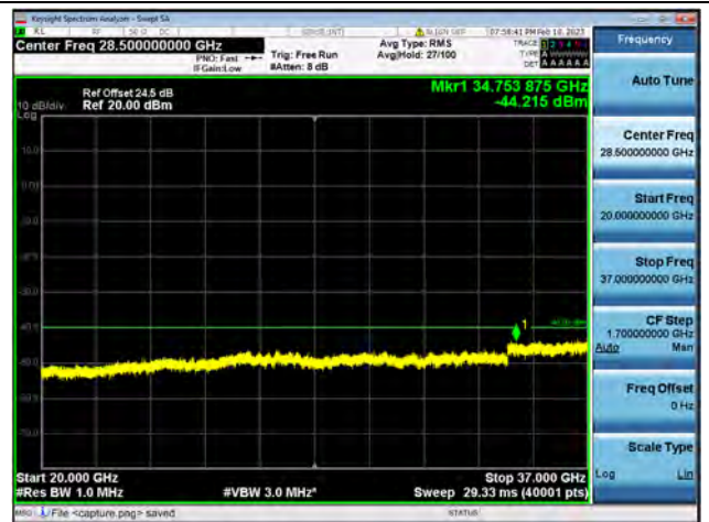
Band48-20G-37G / 20MHz / Low CH / 16QAM
