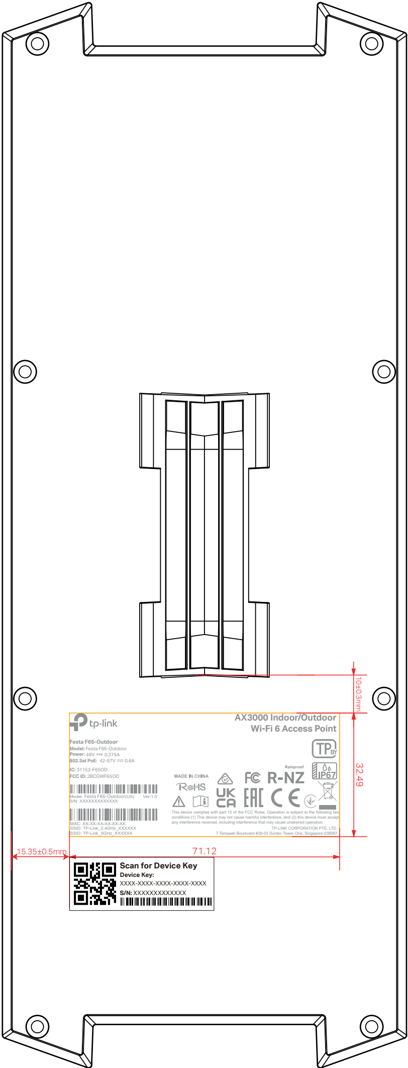
尺寸图
