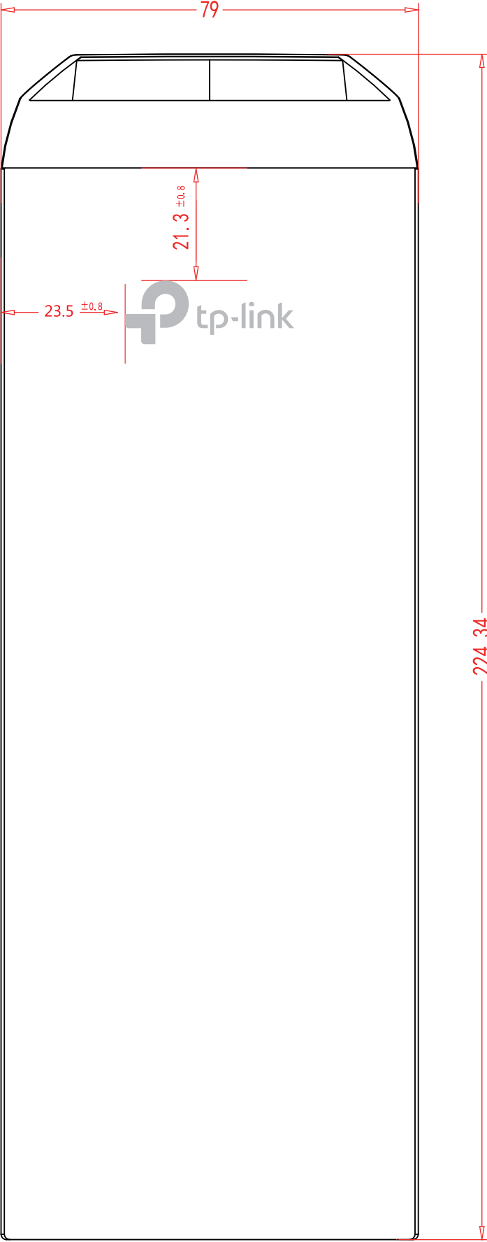
尺寸图
