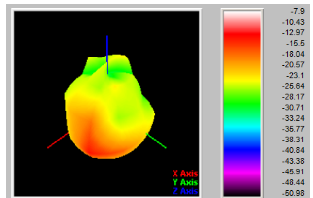
PCS[1900MHz]
