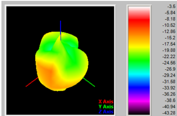
W4[1700MHz]
