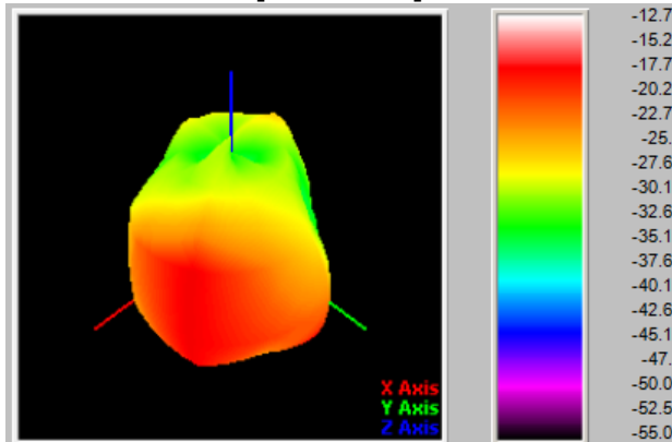
LTEB25[1850MHz]
