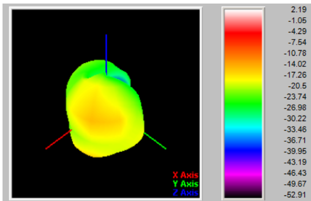
W8[900MHz]
