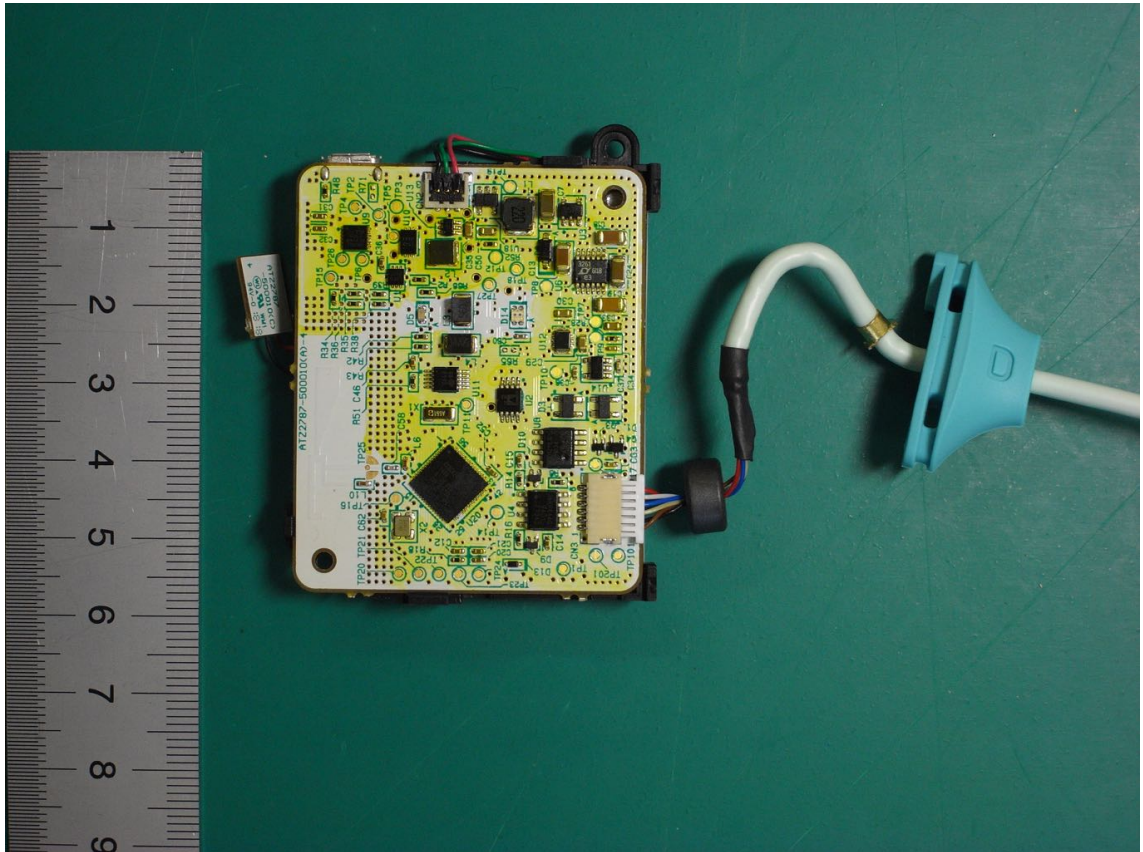
main-front
