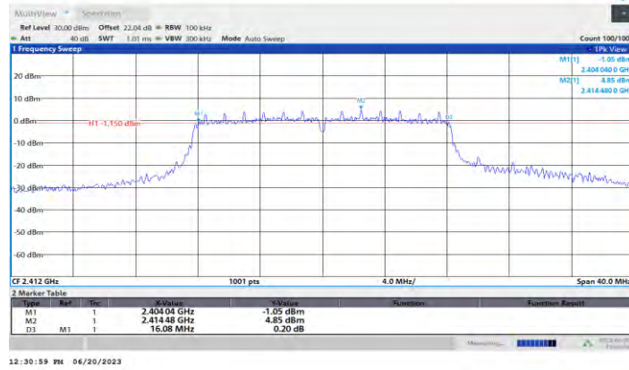
11G_Ant1_2412
