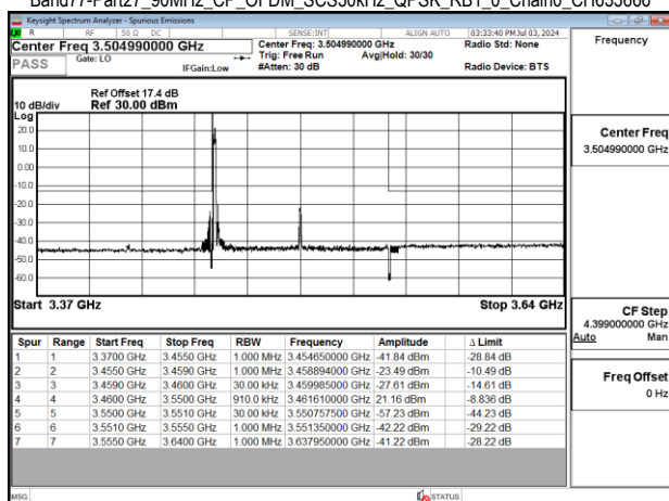
Band77-Part27_90MHz_CP_OFDM_SCS30kHz_QPSK_RB1_0_Chain0_CH633666
