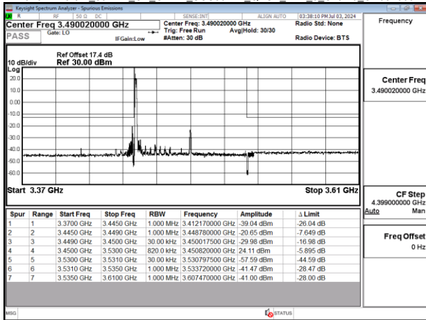
Band77-Part27_80MHz_CP_OFDM_SCS30kHz_QPSK_RB1_0_Chain0_CH633334
