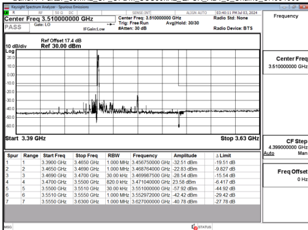
Band77-Part27_80MHz_CP_OFDM_SCS30kHz_QPSK_RB1_0_Chain0_CH634000
