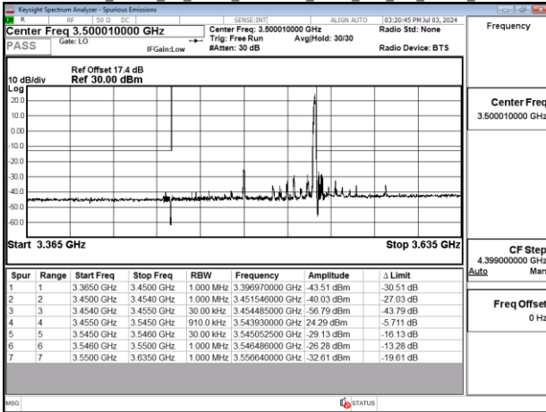
Band77-Part27_90MHz_CP_OFDM_SCS30kHz_QPSK_RB1_244_Chain0_CH633666
