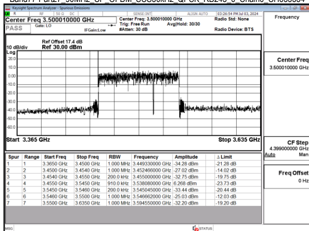
Band77-Part27_90MHz_CP_OFDM_SCS30kHz_QPSK_RB245_0_Chain0_CH633666
