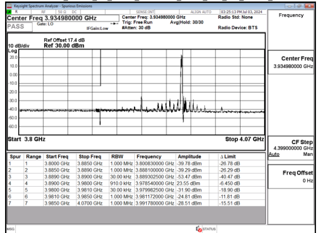
Band77-Part27_90MHz_CP_OFDM_SCS30kHz_QPSK_RB1_244_Chain0_CH62332
