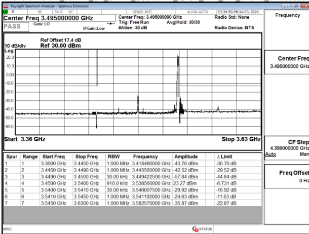
Band77-Part27_90MHz_CP_OFDM_SCS30kHz_QPSK_RB1_244_Chain0_CH633334
