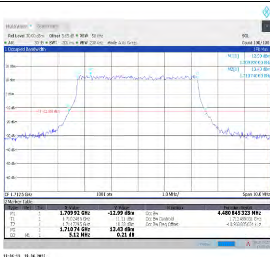
1-N66-PC3-15-5-L-1-DFT-QPSK-Outer_Full-25@0-A nt1-4.481-5.120-≤5-PASS
