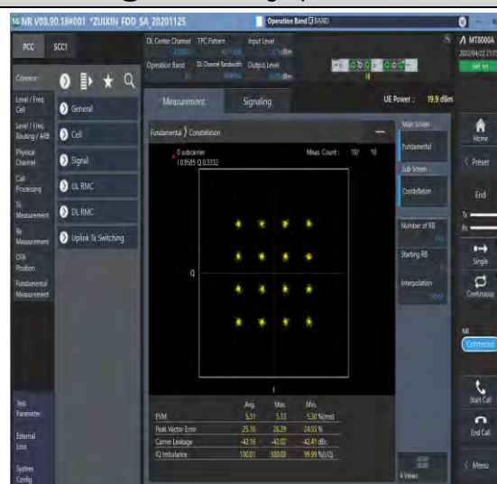
1-N66-PC3-15-40-M-7-CP-16QAM-Outer_Full-216@ 0-Ant1-see graph-PASS
