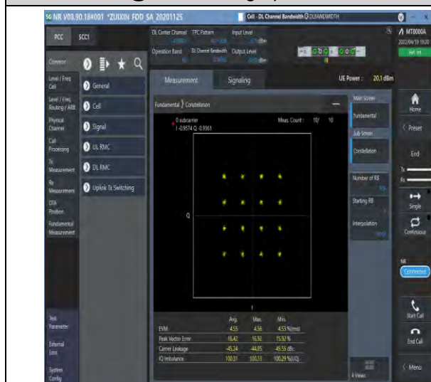
1-N66-PC3-15-20-M-7-CP-16QAM-Outer_Full-106@ 0-Ant1-see graph-PASS
