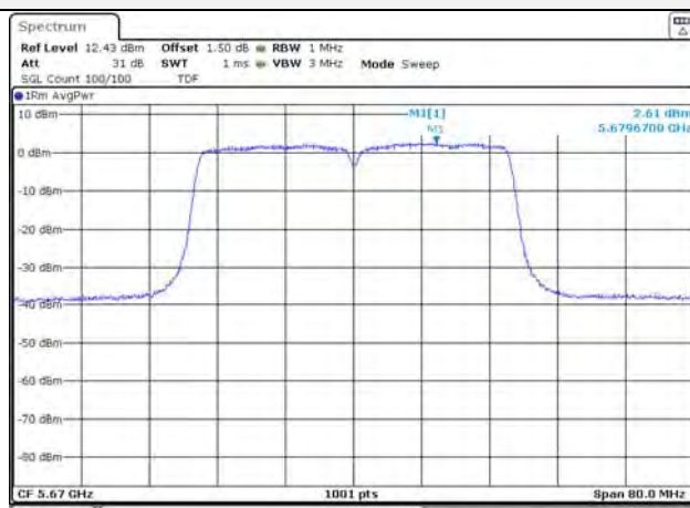
UNII-2C / 802.11ac VHT40 / 5 670 MHz
