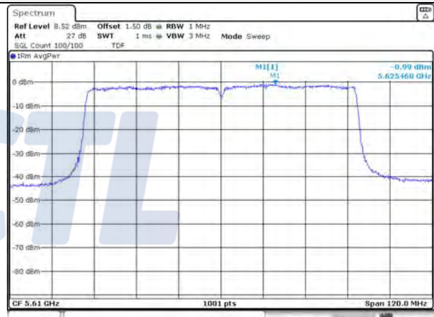
UNII-2C / 802.11ac VHT80 / 5 610 MHz
