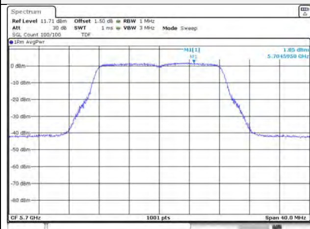
UNII-2C / 802.11a / 5 700 MHz
