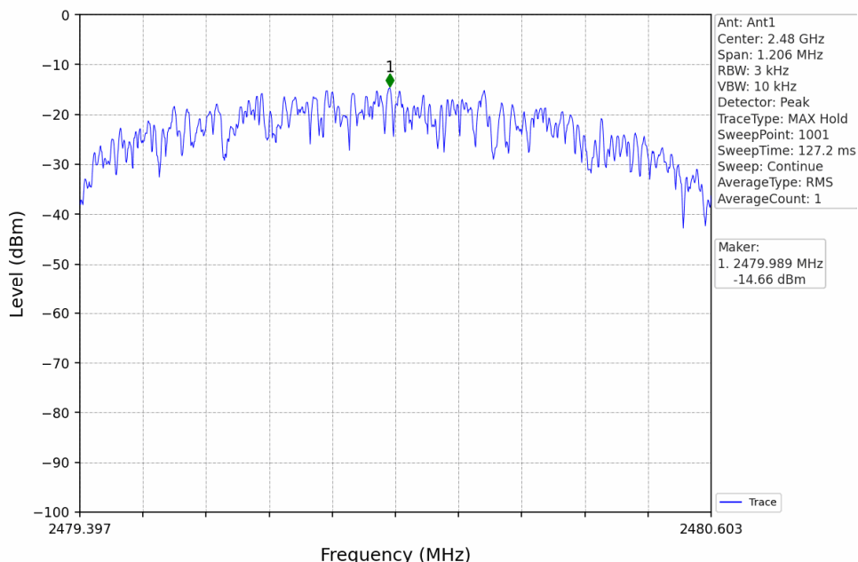
1M_HCH_2480MHz_DataRate=_Ant1_NTNV
