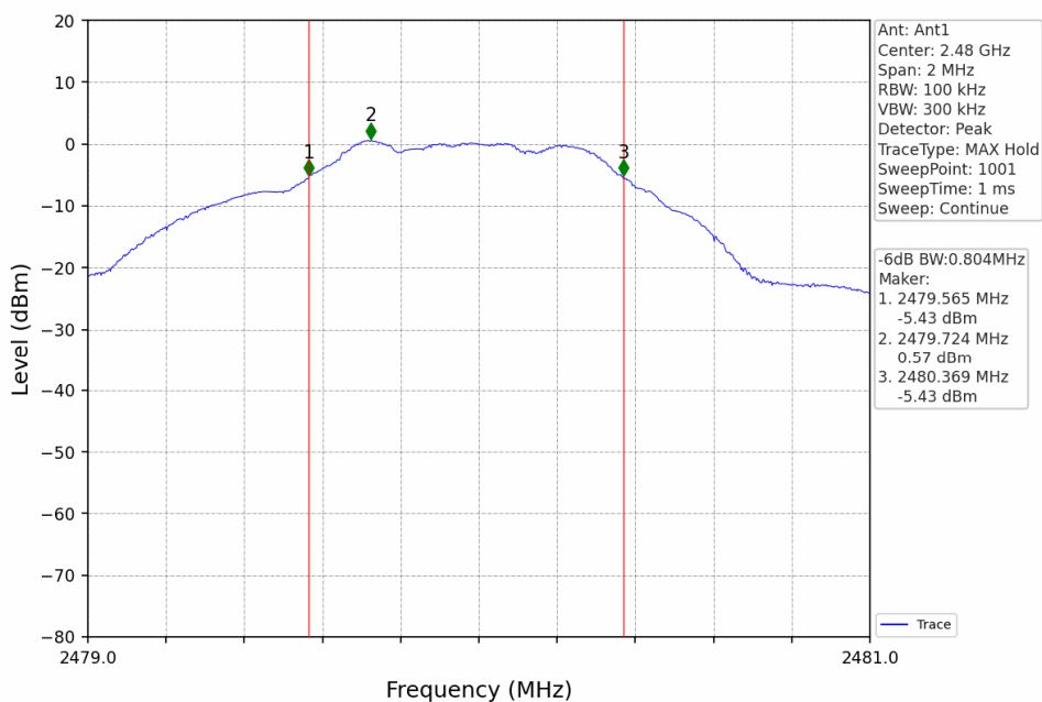
1M_HCH_2480MHz_DataRate=_Ant1_NTNV
