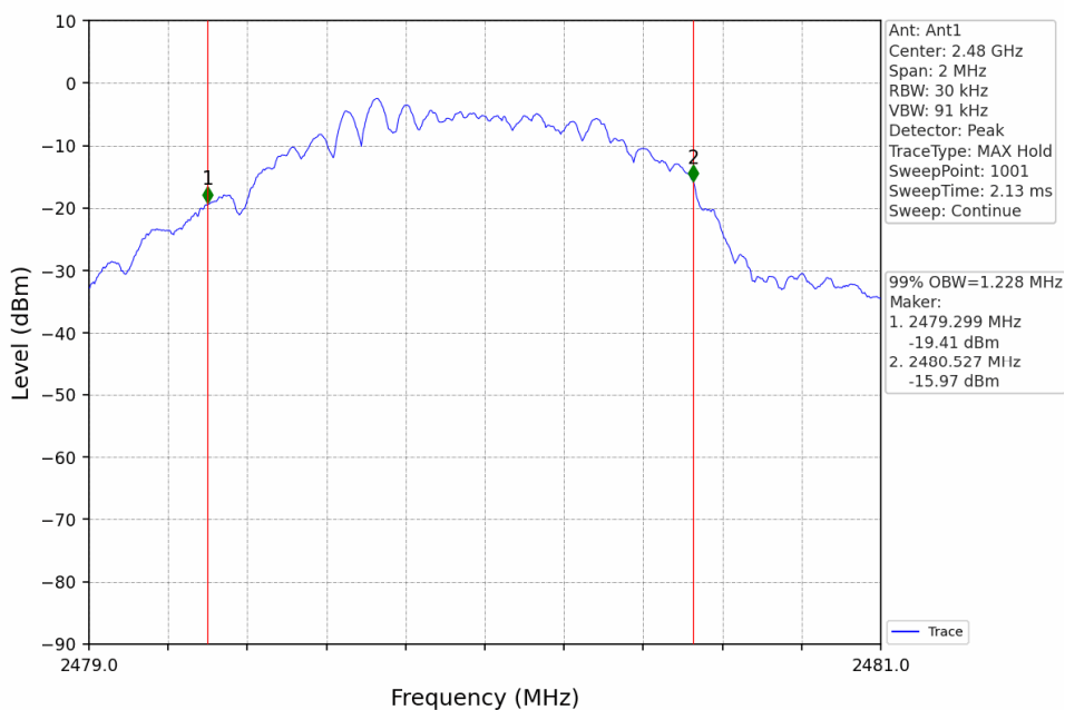
1M_HCH_2480MHz_DataRate=_Ant1_NTNV
