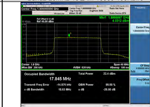
Band2-20MHz-16QAM-19100-100RB#0
