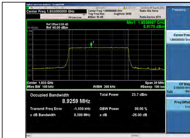
Band2-10MHz-QPSK-18650-50RB#0
