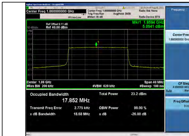
Band2-20MHz-QPSK-18700-100RB#0
