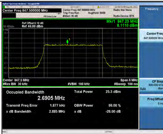
Band5-3MHz-QPSK-20635-15RB#0
