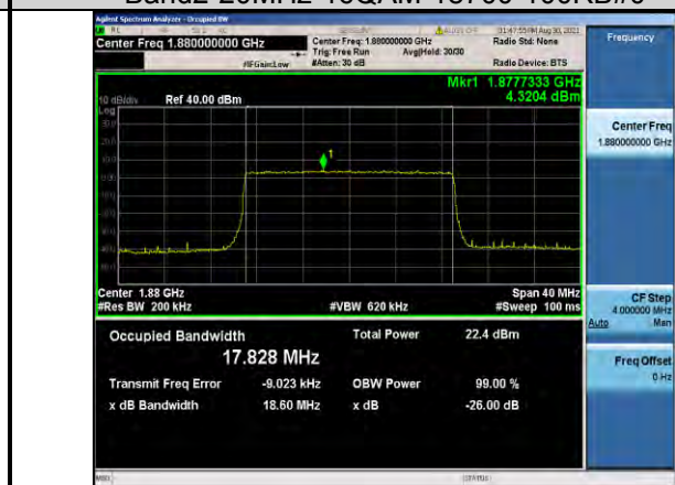
Band2-20MHz-16QAM-18900-100RB#0
