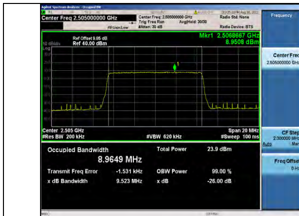
Band7-10MHz-QPSK-20800-50RB#0
