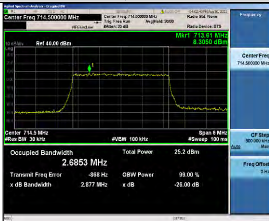
Band12-3MHz-QPSK-23165-15RB#0
