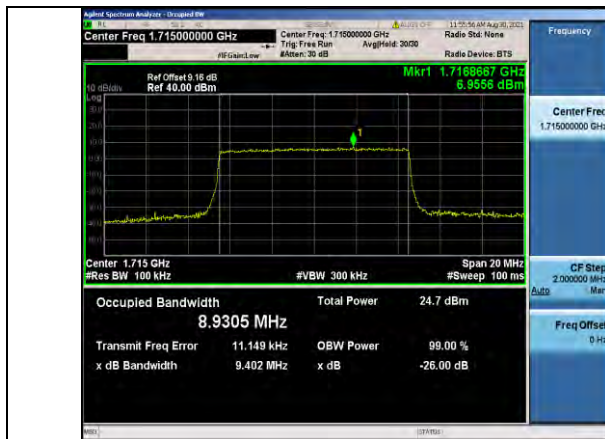
Band4-10MHz-QPSK-20000-50RB#0
