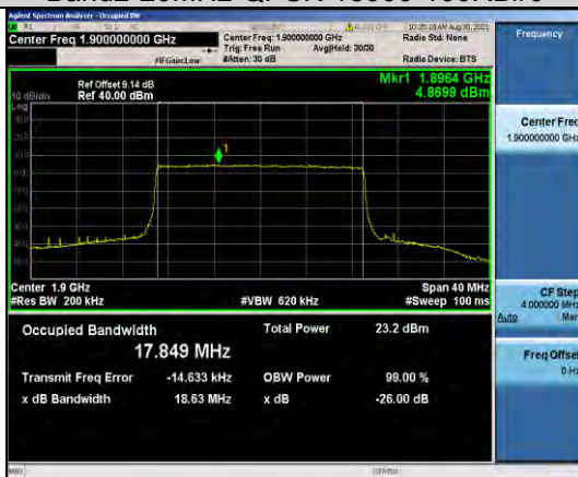
Band2-20MHz-QPSK-19100-100RB#0
