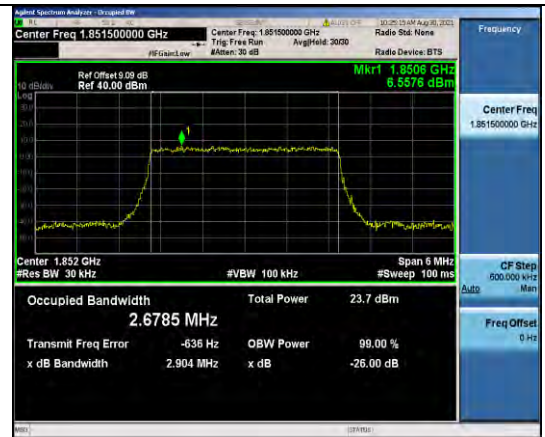
Band2-3MHz-16QAM-18615-15RB#0
