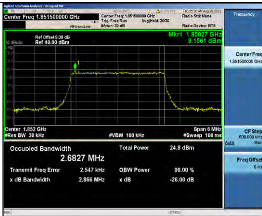
Band2-3MHz-QPSK-18615-15RB#0
