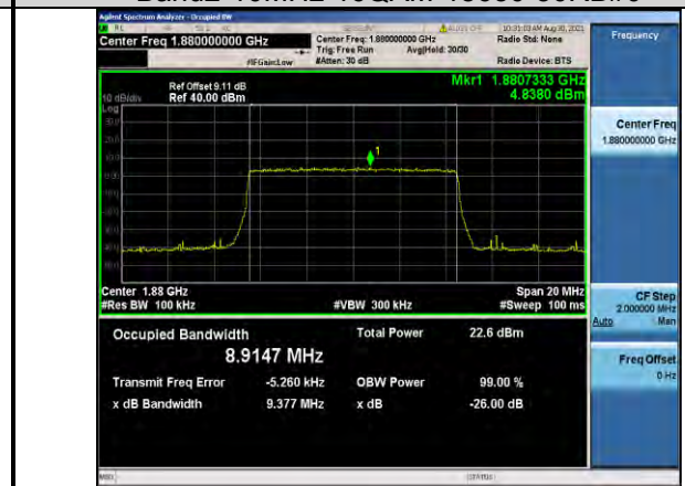
Band2-10MHz-16QAM-18800-50RB#0
