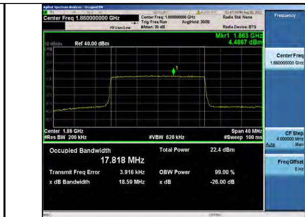
Band2-20MHz-16QAM-18700-100RB#0
