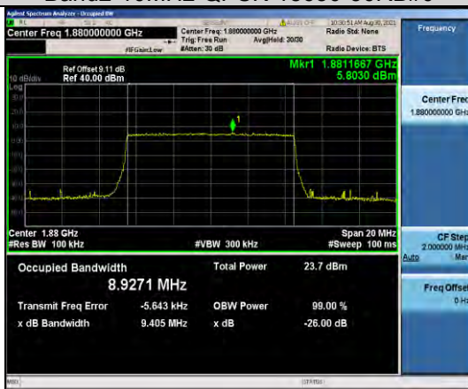
Band2-10MHz-QPSK-18800-50RB#0
