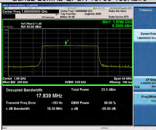
Band2-20MHz-QPSK-18900-100RB#0
