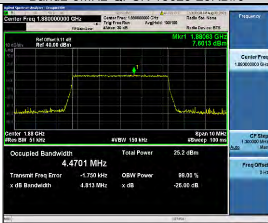
Band2-5MHz-QPSK-18900-25RB#0
