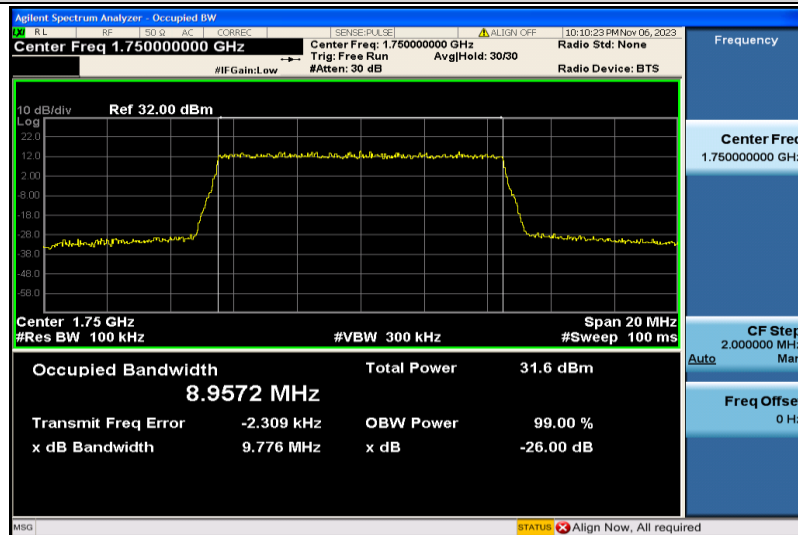
Band4-10MHz-QPSK-20350-50RB#0-8.9572
