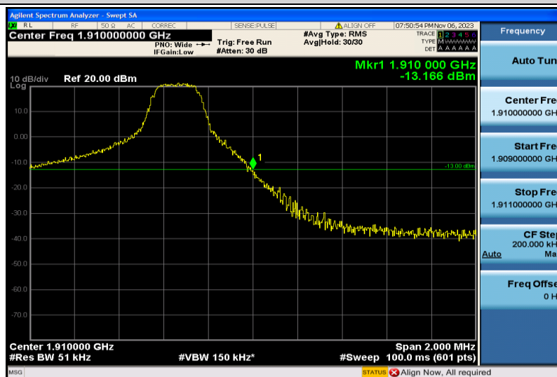
Band2-5MHz-QPSK-19175-1RB#24
