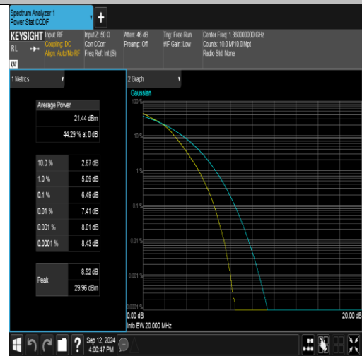
Band2-20MHz-16QAM-18700-100RB#0-PASS
