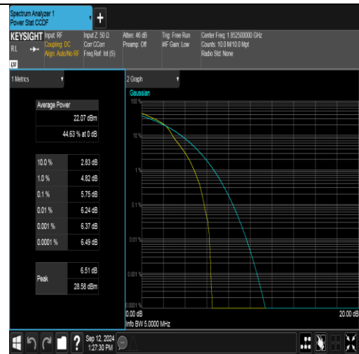
Band2-5MHz-16QAM-18625-1RB#0-PASS
