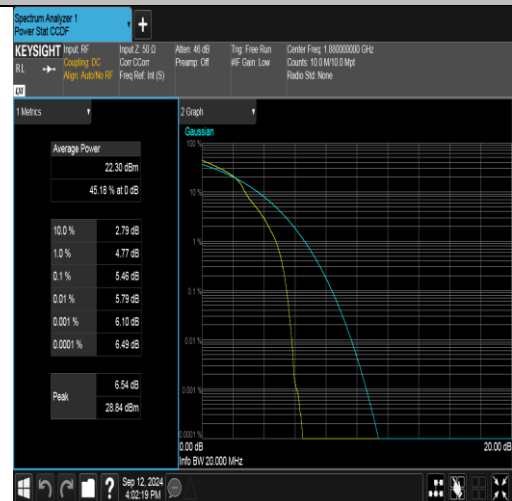
Band2-20MHz-16QAM-18900-1RB#0-PASS
