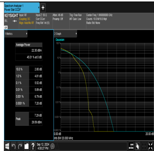
Band2-20MHz-16QAM-18700-1RB#0-PASS
