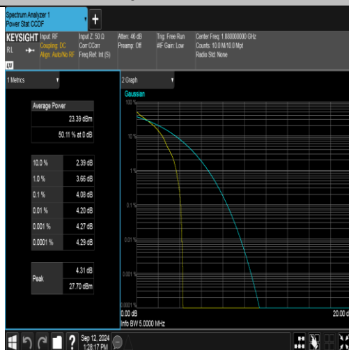
Band2-5MHz-QPSK-18900-1RB#0-PASS
