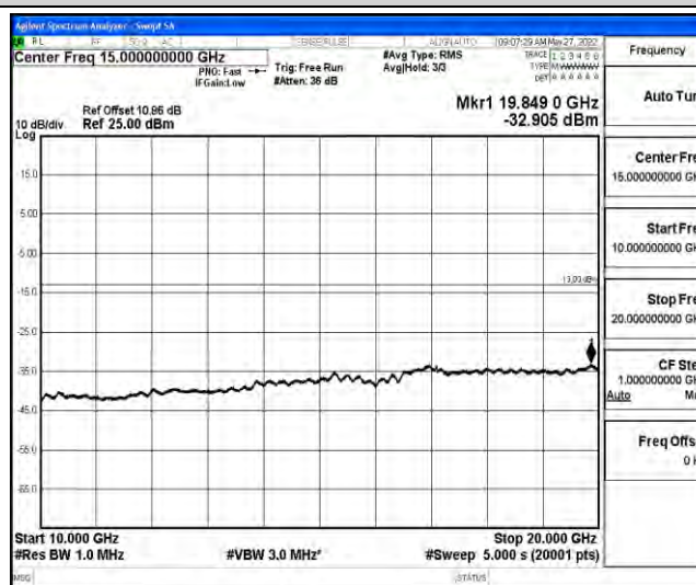
Band2-20MHz-QPSK-18700-1RB#0-Range5:10000~20000MHz
